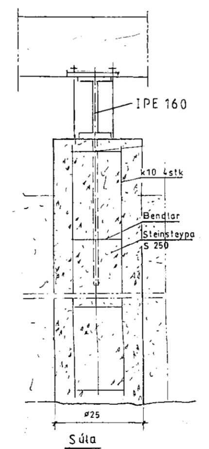
Snid A-A Mkv=1:10
