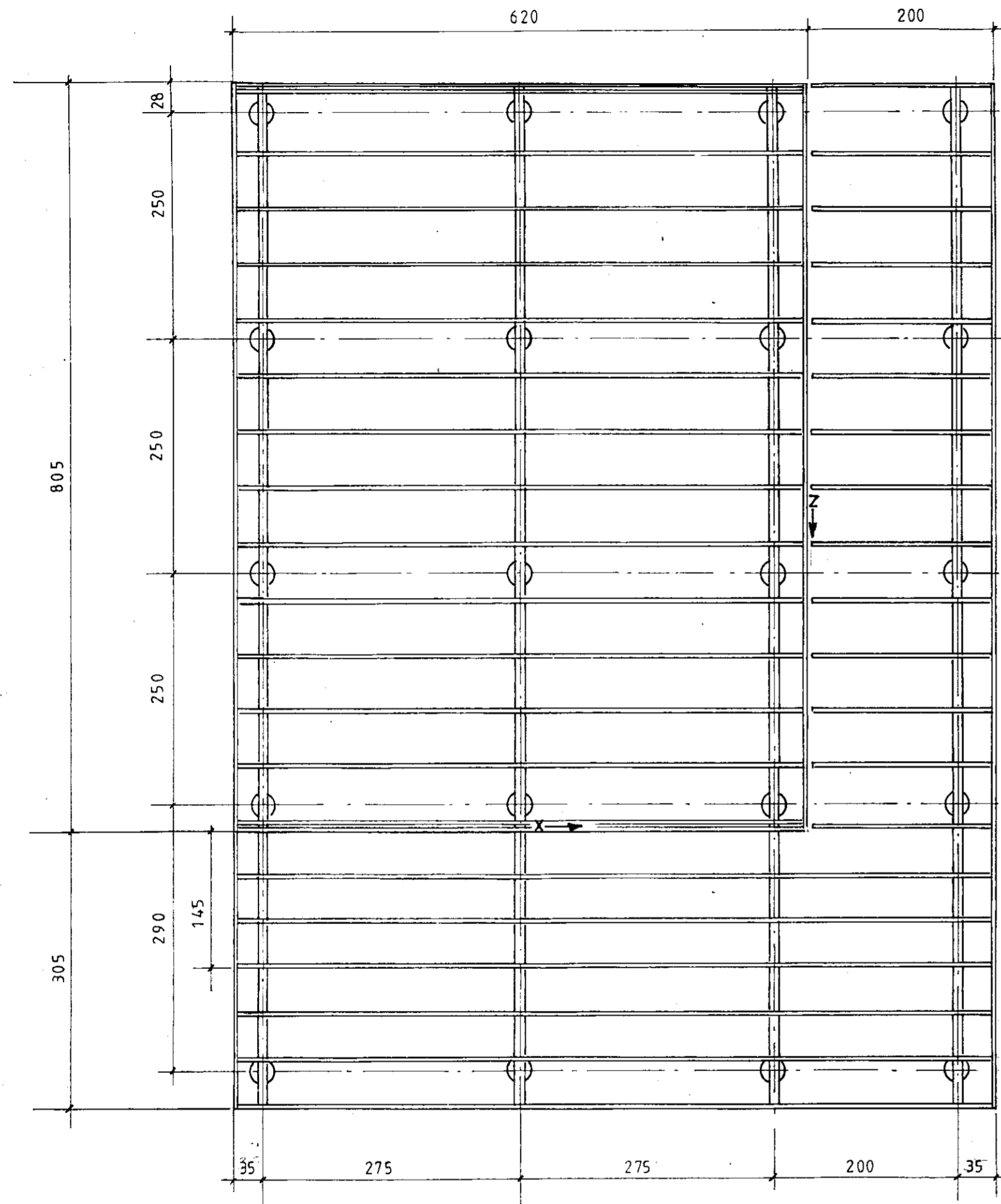
Undirstödur og gólf Mkv 1:50
