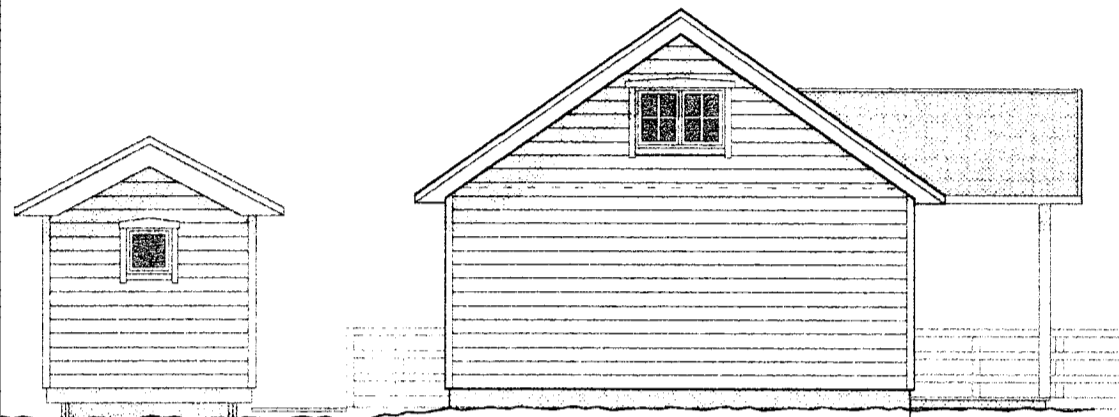
ÚTLIT NORÐUR
