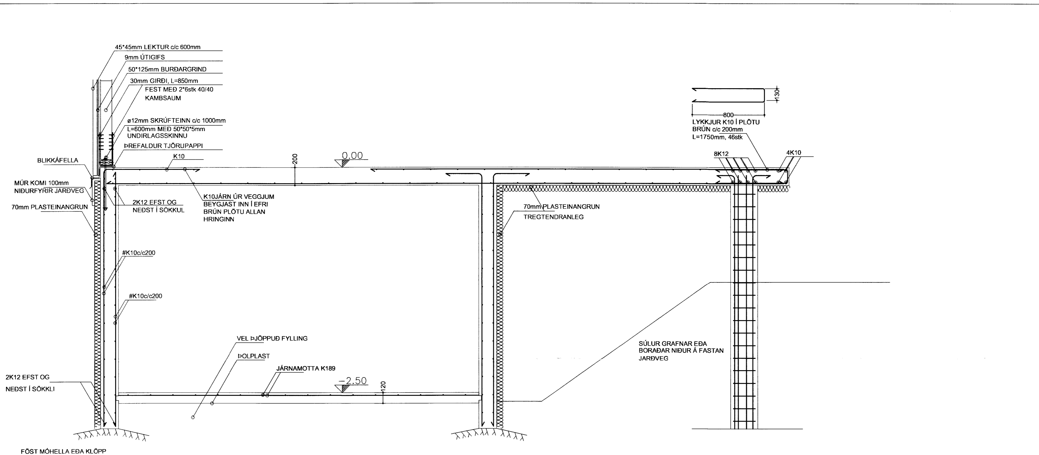
A 300/100 SNEIÐING mkv. 1:20
