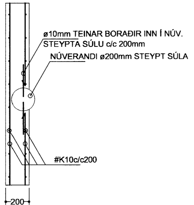
C 300/100 SNEIÐING mkv. 1:20
