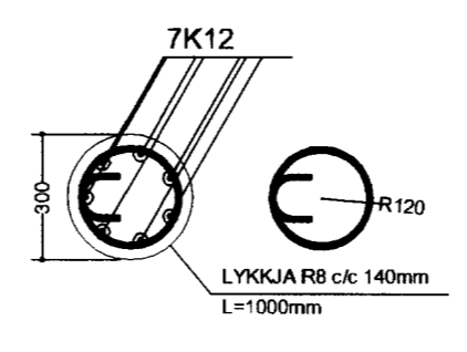
D 300/100 SNEIÐING mkv. 1:20
