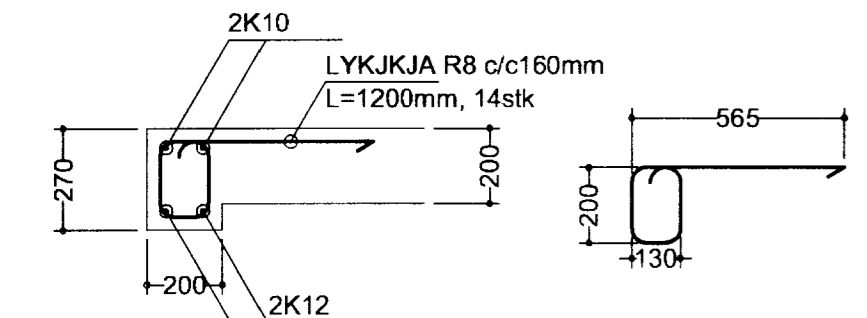
B 300/100 SNEIÐING mkv. 1:20
