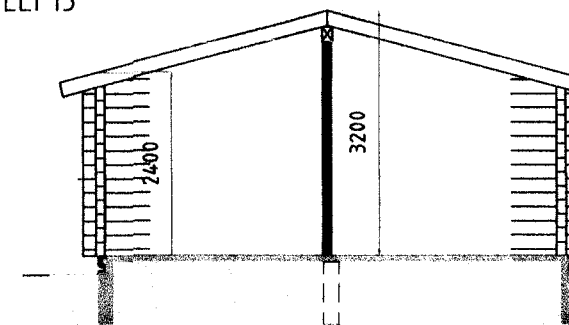
SNEIÐMYND A-A
