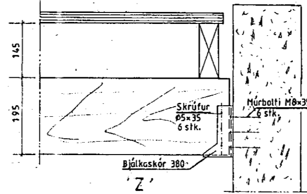
Binding verandar við sökkul og sútu
