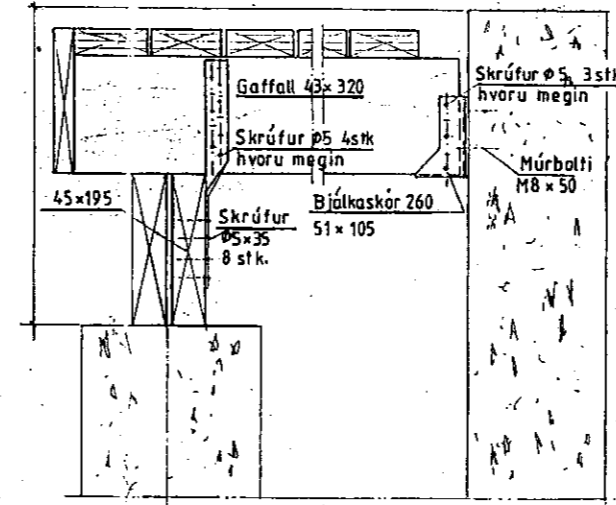
Binding verandar við sökkul og sútu
