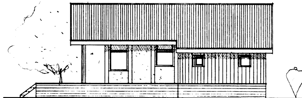
AUSTURHLIÐ MKV. 1:100.
