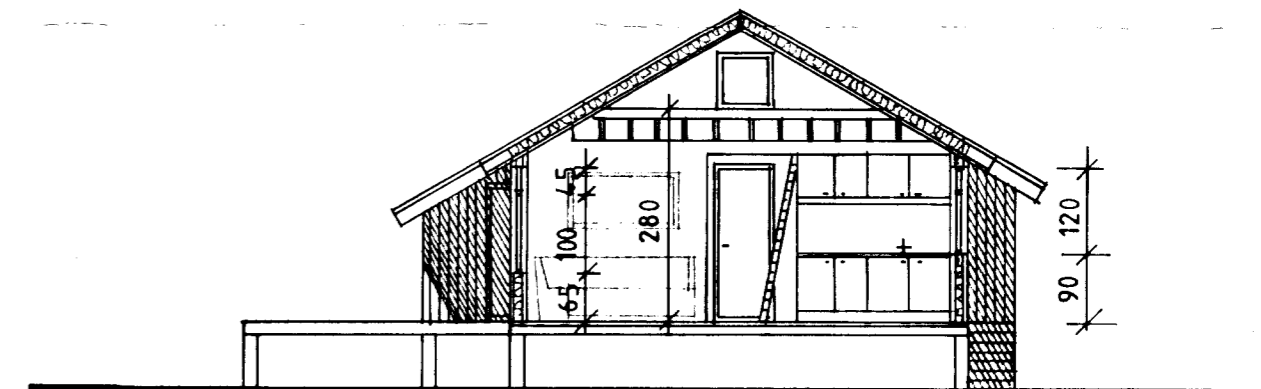
SNEIÐING B-B. MKV. 1:100.
