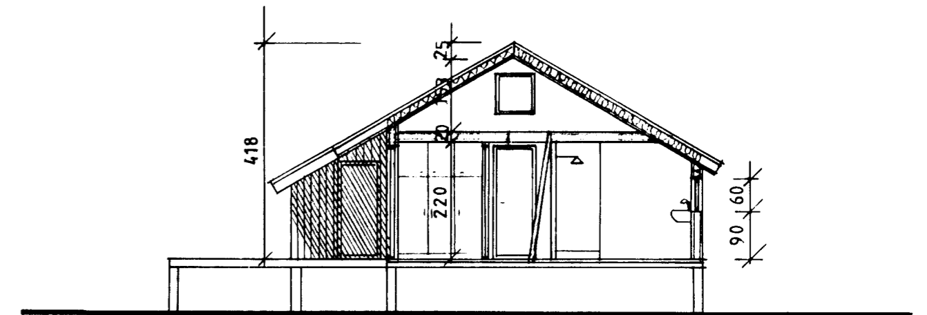
SNEIÐING A-A. MKV. 1:100.
