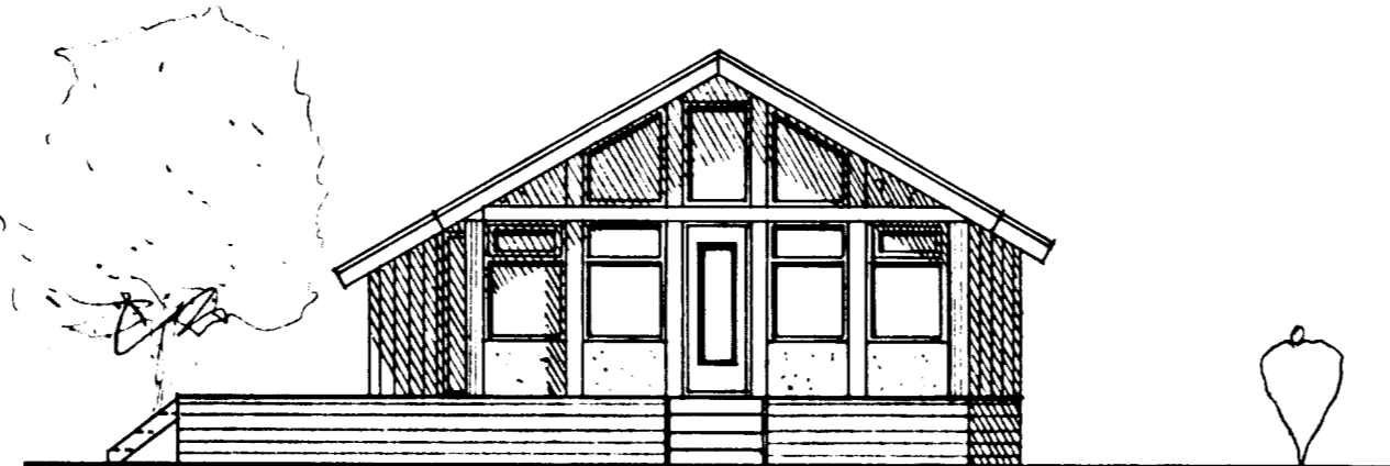
SUÐURHLIÐ MKV. 1:100.
