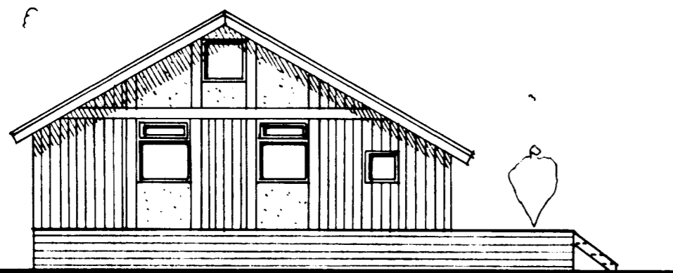
NORÐURHLIÐ MKV. 1:100
