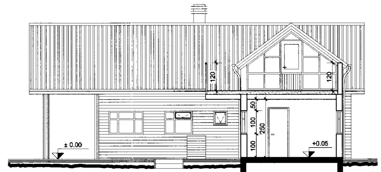
Snið B-B
