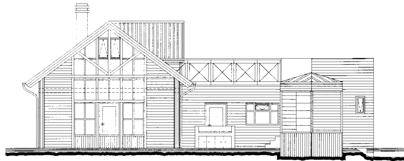
Norðurhlið
