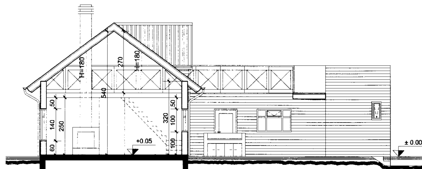
Snið A-A
