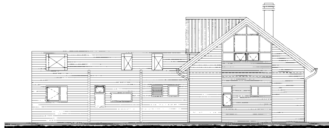
Suðurhlið
