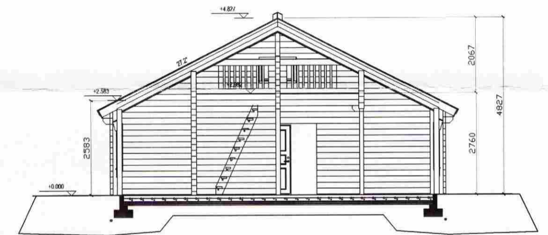
SNID A-A
