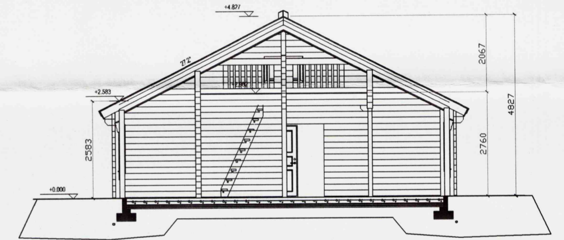
SNID A-A
