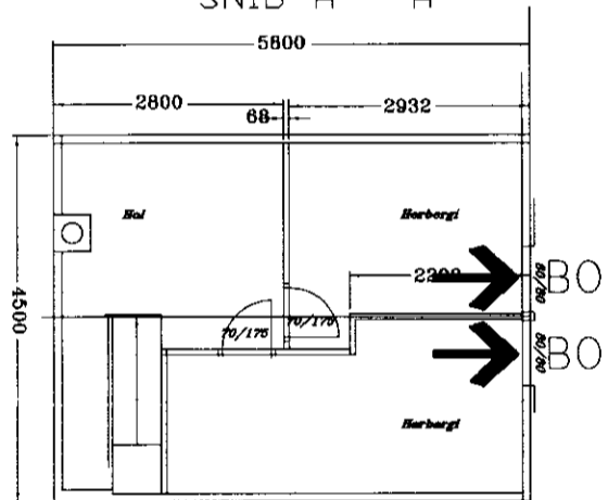
SVEFNLOFT
