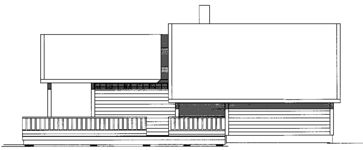
AUSTUR
