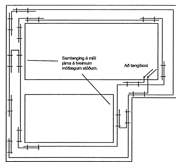
Grunnmynd sökkulveggja
