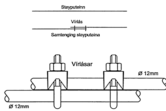
Samtenging steypusteinna
