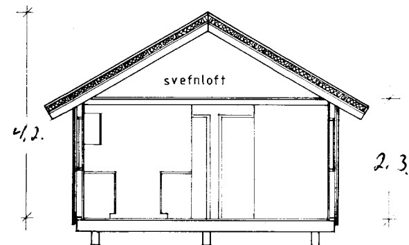
SKURDUR A-A
