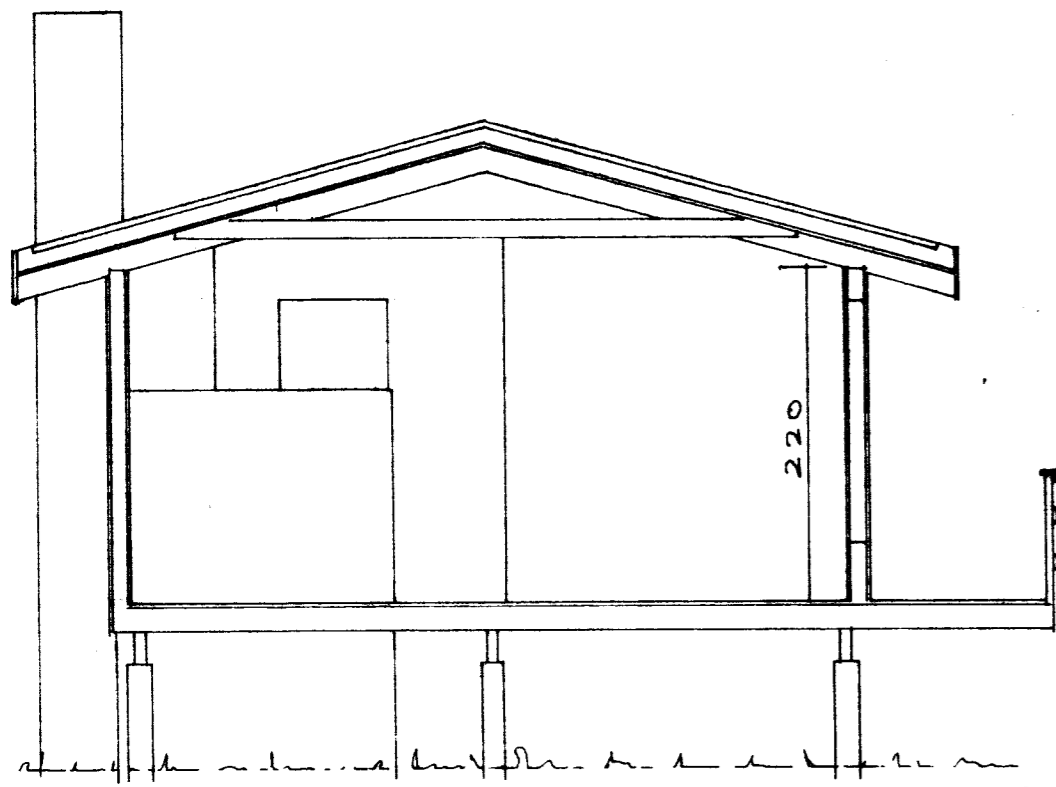
skurður A-A
