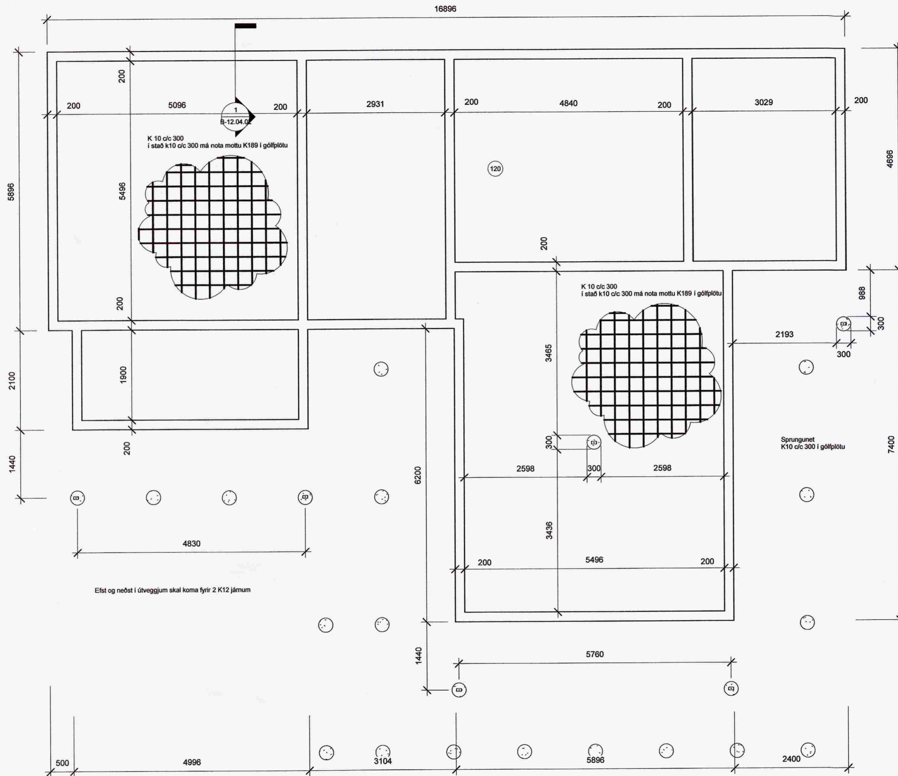
1 Undirstöður 1 : 50
