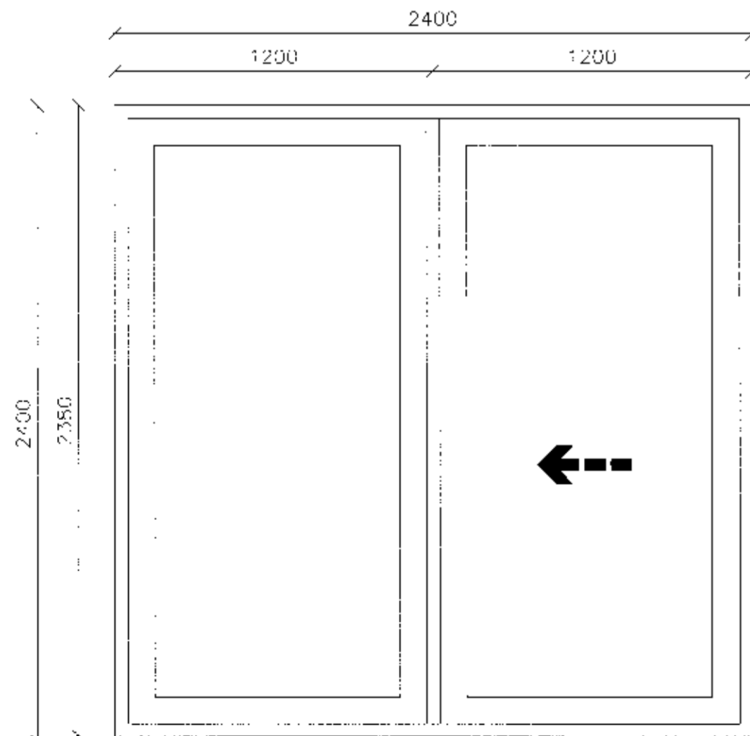
H-1 Hæð ofan á glugga.....2400mm Rennihurð Fjöldi .....2.stk.
