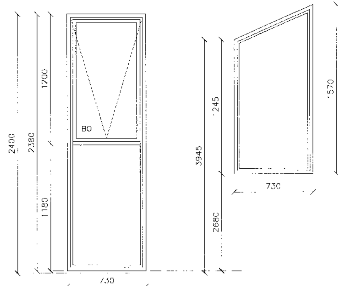
G-7 Hæð ofan á glugga.....2400mm Opnanlegt fag.....Toppengt Fjöldi .....2.stk.
