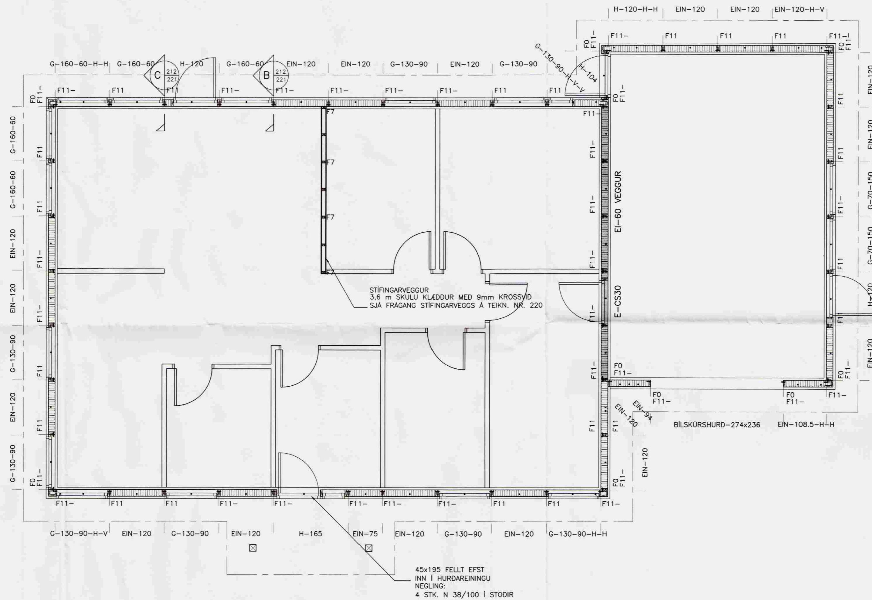
VEGGJAPLAN MKV. 1:50
