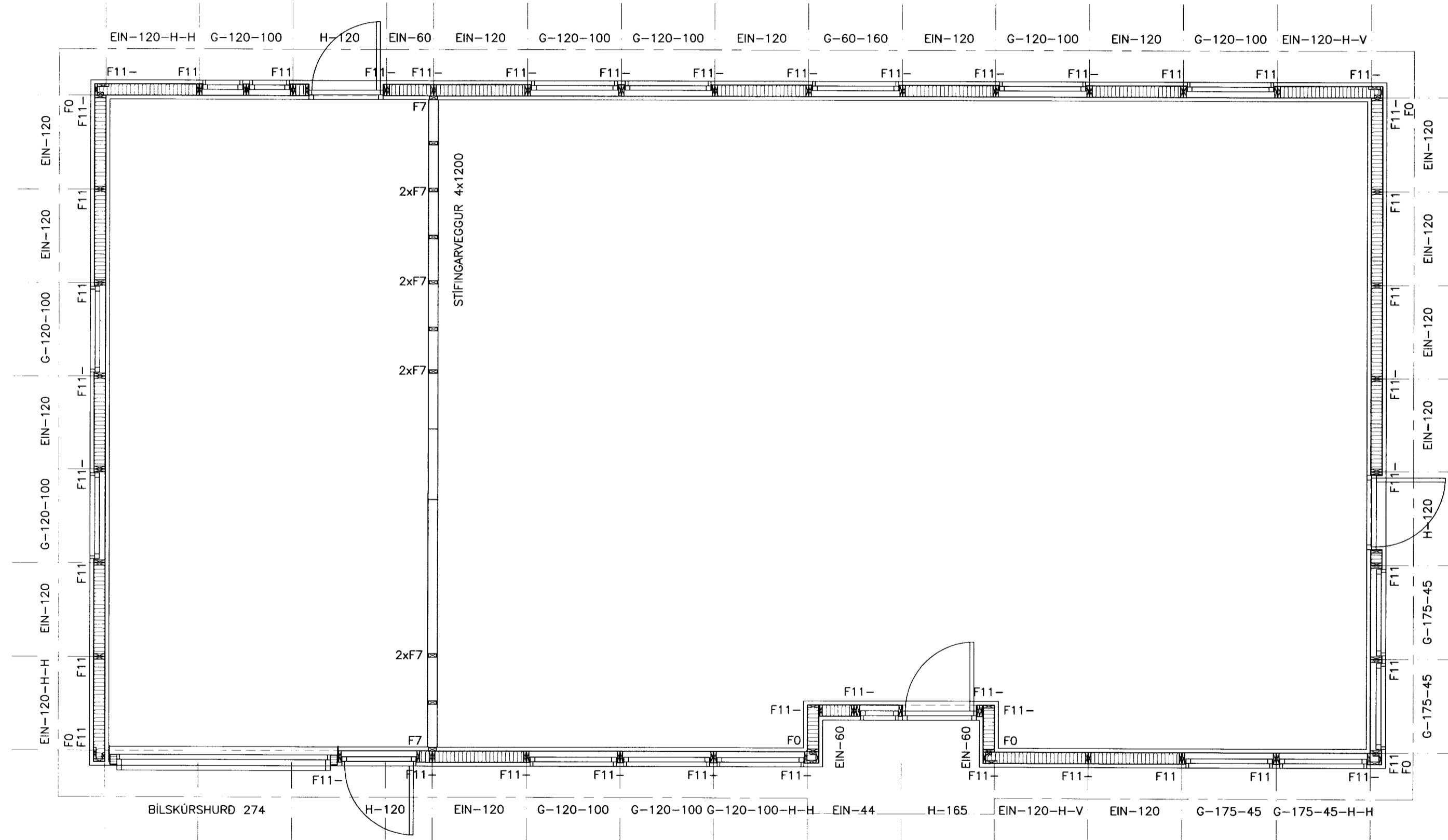
VEGGJAPLAN Mkv. 1:50
