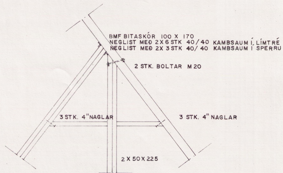
D 3 M D3. MKV. 1:20
