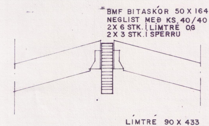
SNÍÐ A-A MKV. 1:20
