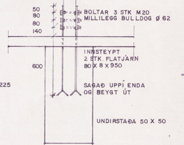
FRÁGANGUR VIÐ SÚLUR
