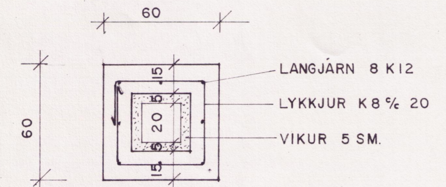
SKORSTEINN MKV. 1:20
