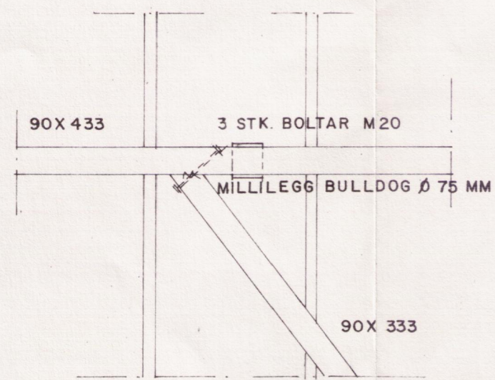
D4 MKV. 1:20
