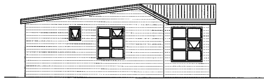
ÚTLIT NORÐUR mkv. 1:100
