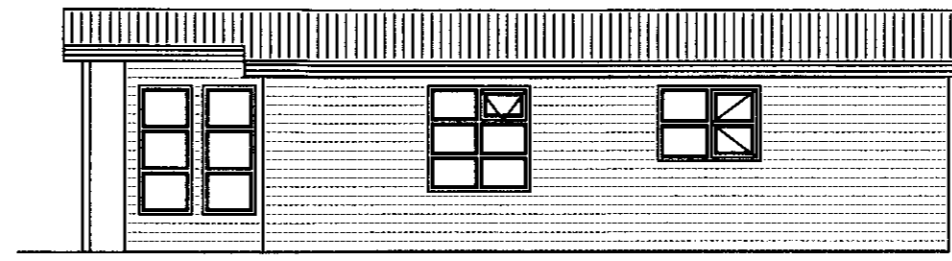
ÚTLIT AUSTUR mkv. 1:100
