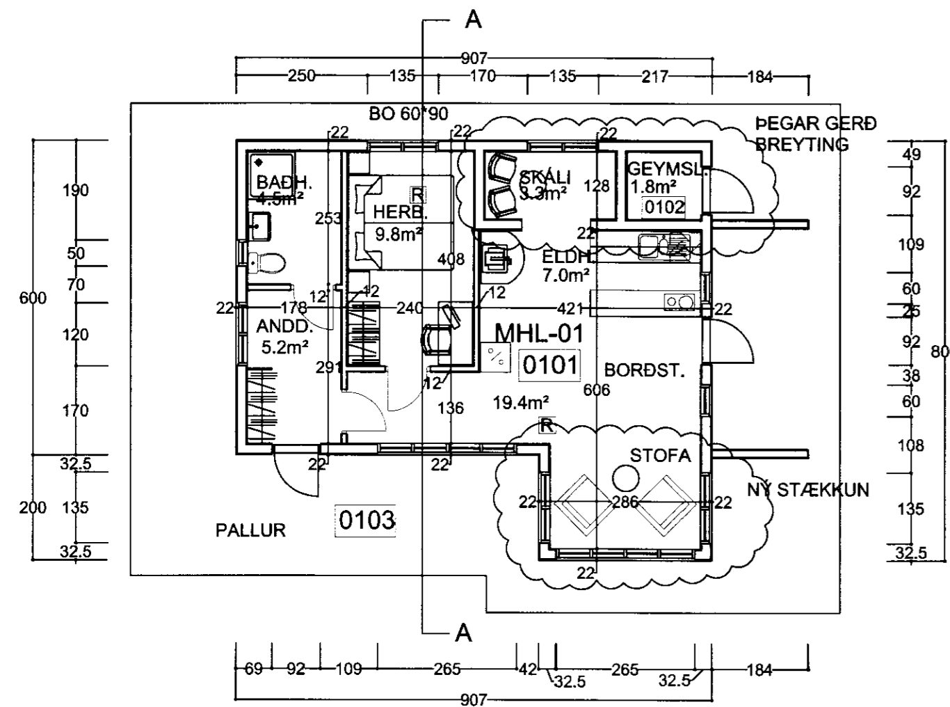
GRUNNMYND, mkv. 1:100
