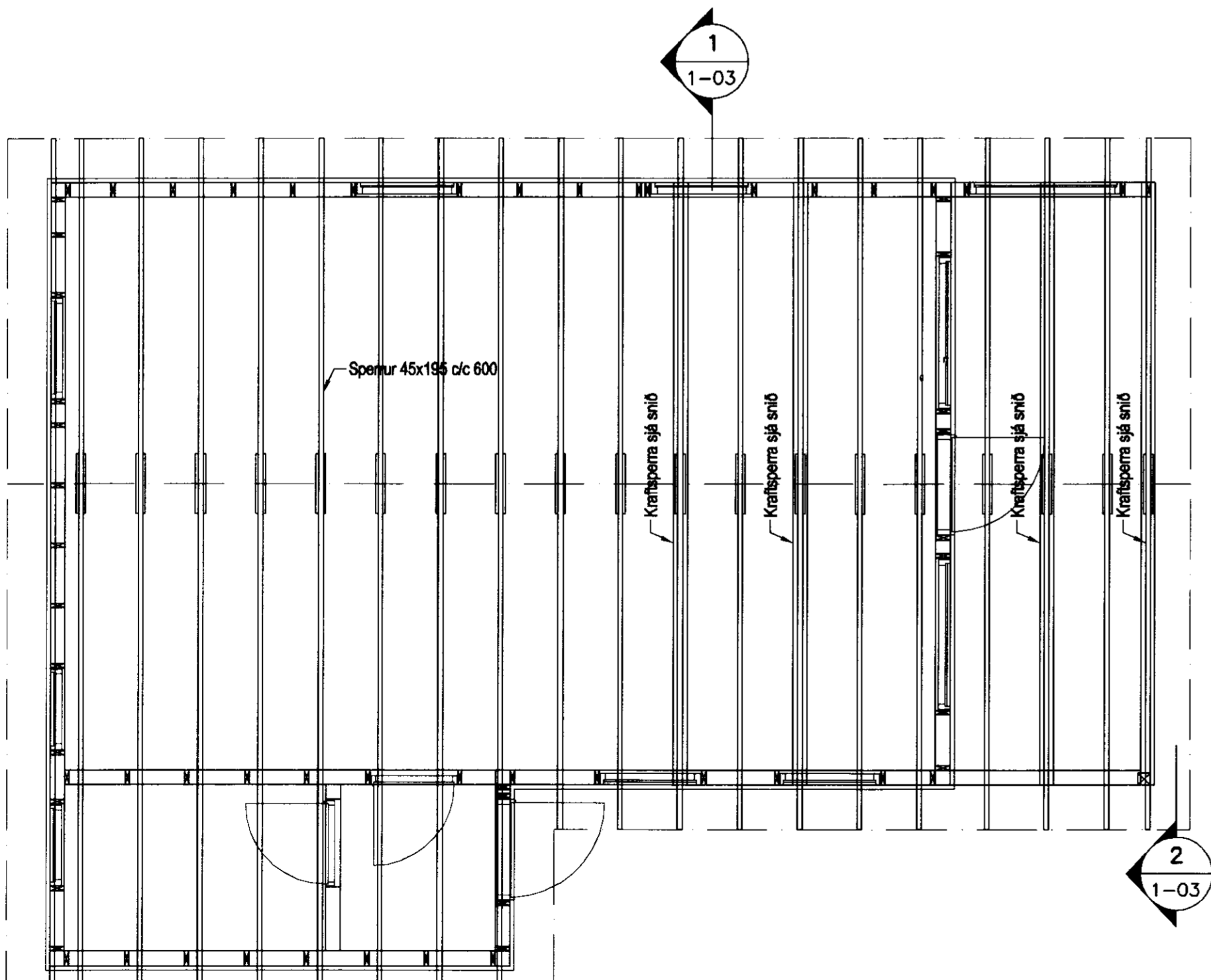
Grunnmynd, 1:50
