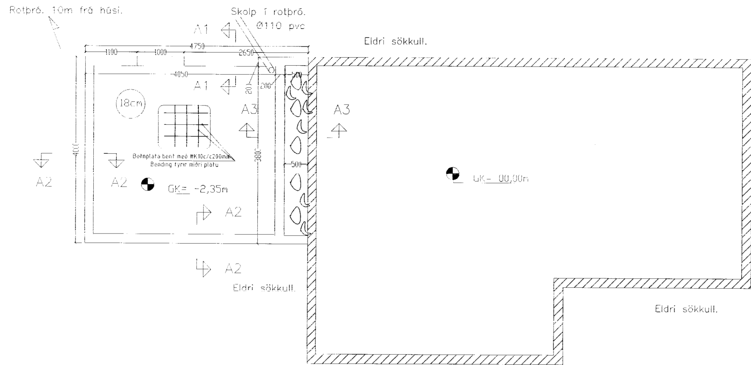
Grunnmynd sökla 1:50
