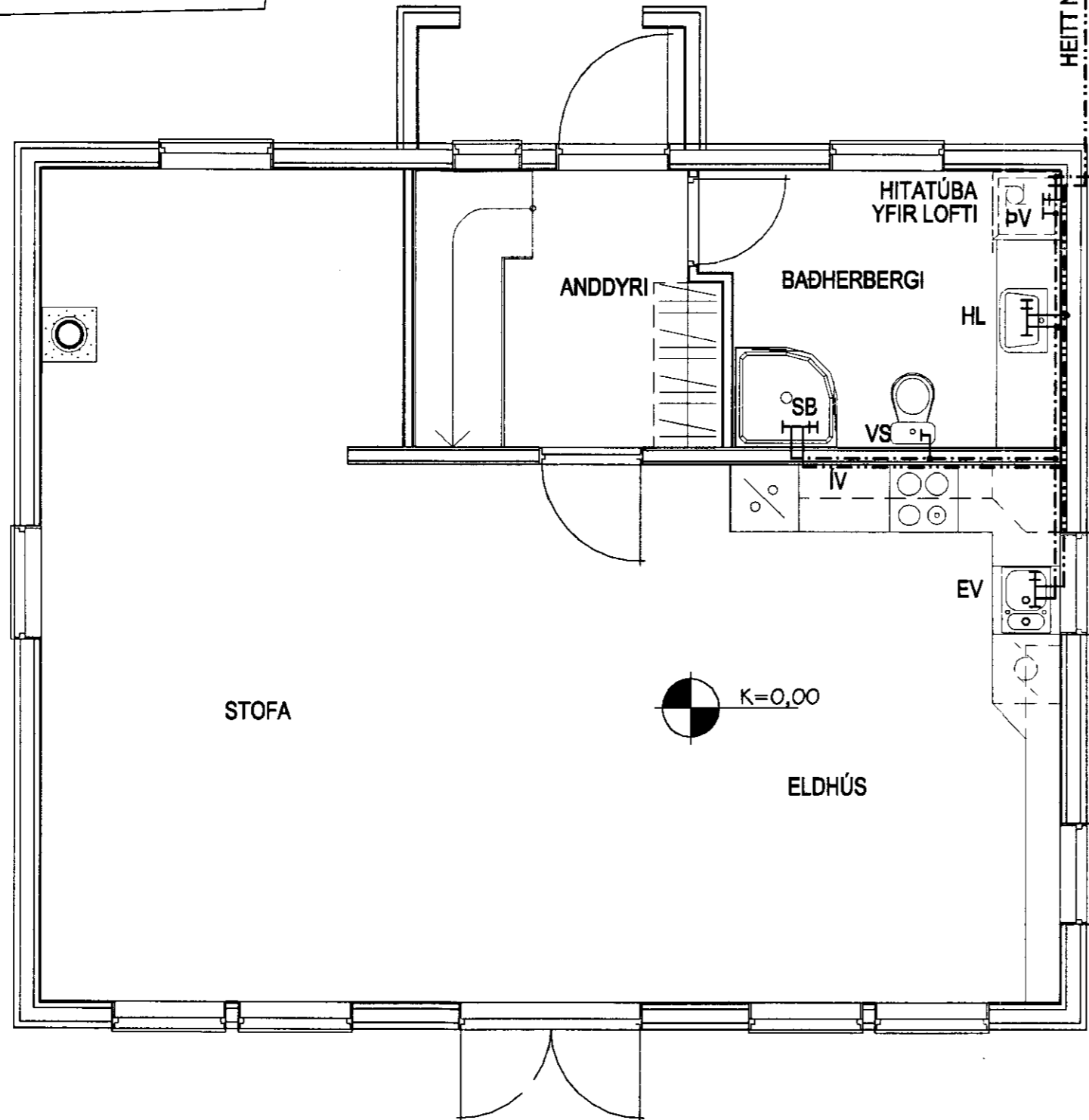
NEYSLUVATNSLAGNIR, GRUNNMYND NEDRI HÆÐAR MKV. 1:50
