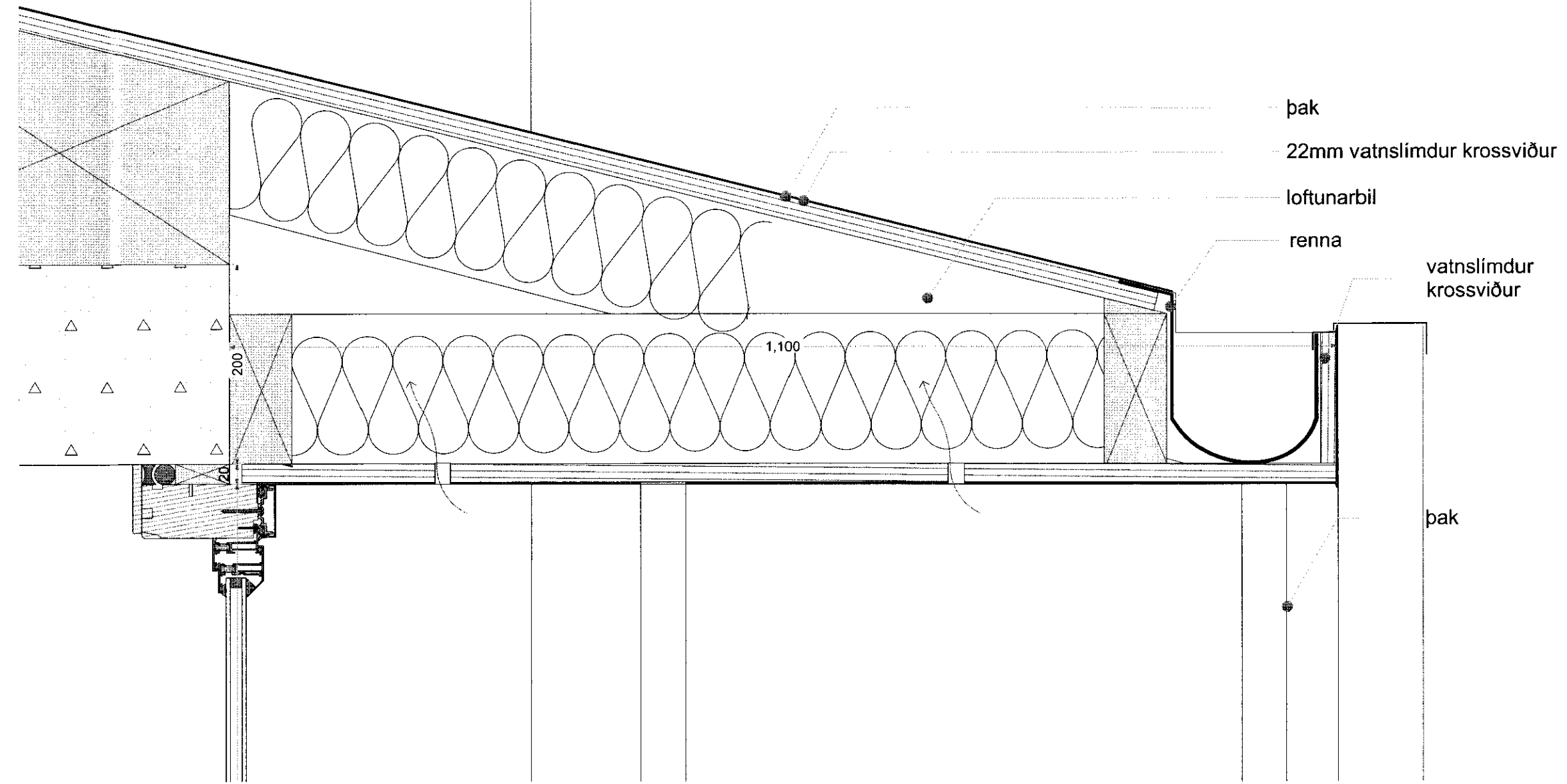
S-12 Þakkantur 1:5
