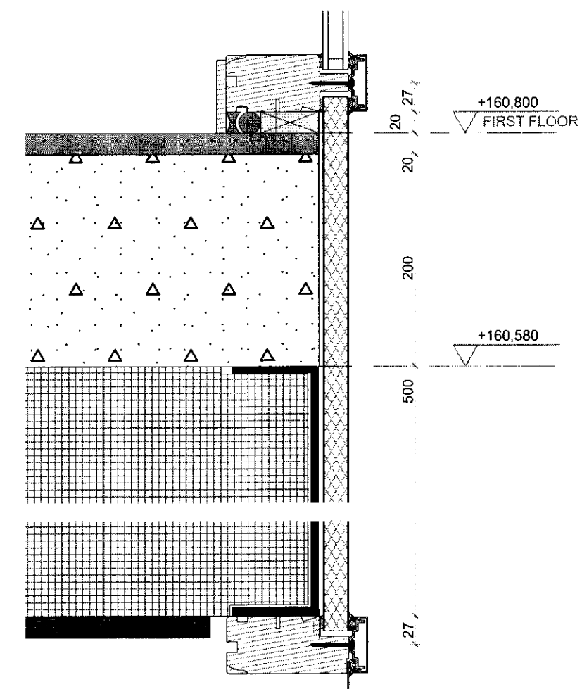
D-03 Deilal 1:5
