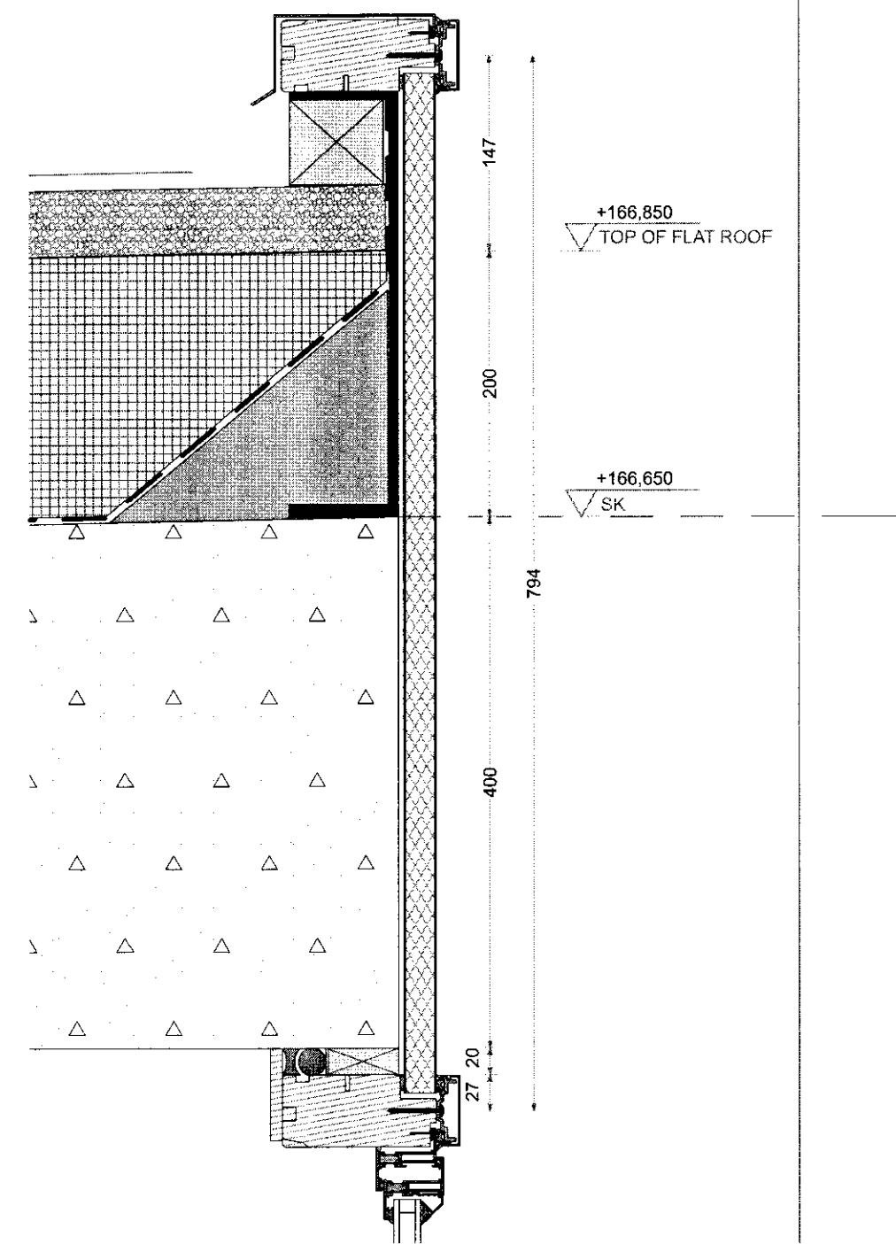
D-01 Deilal 1:5
