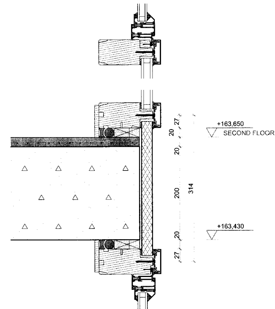
D-02 Deilal 1:5
