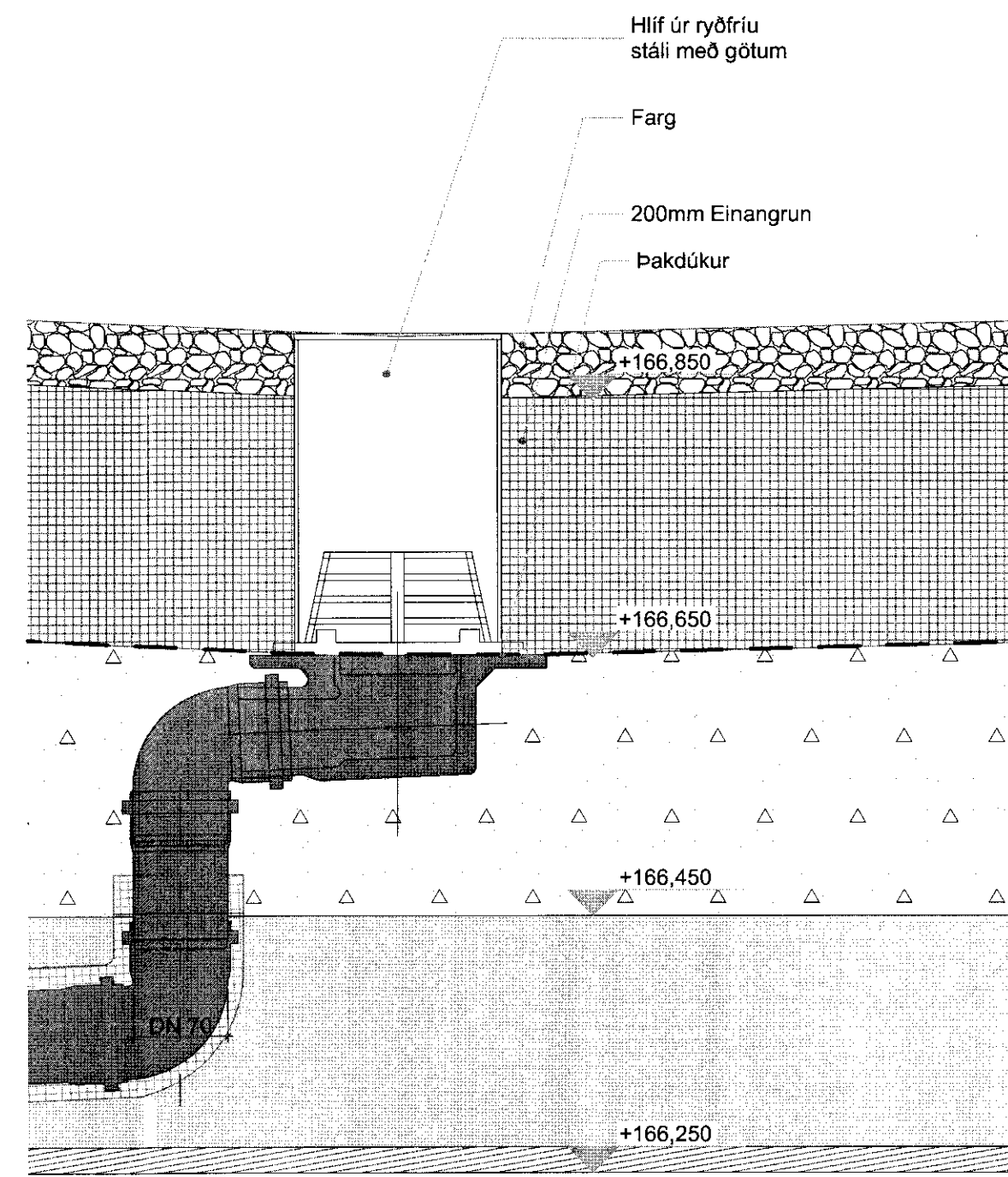
D-04 Deilal 1:5
