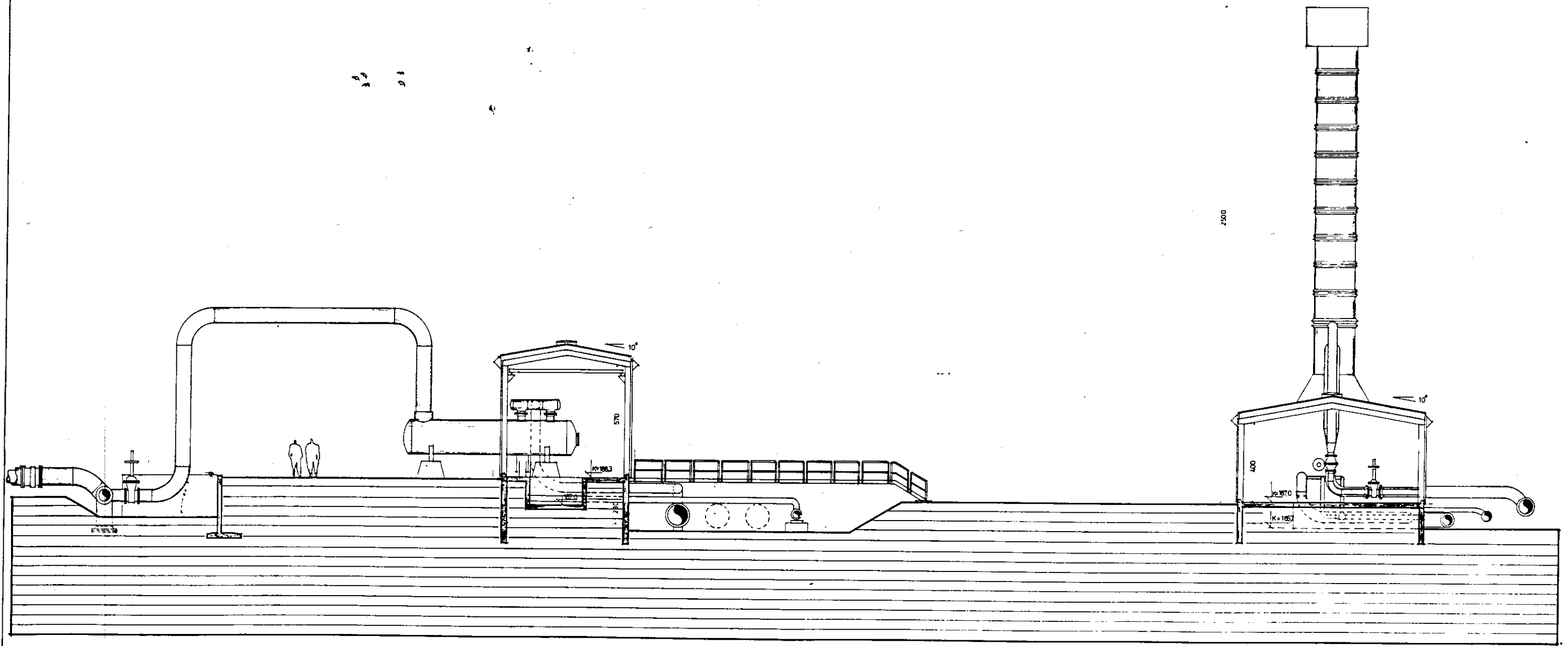
sneiding A-A
