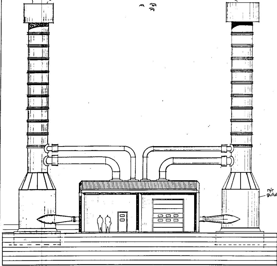
útlit nord-vestur
