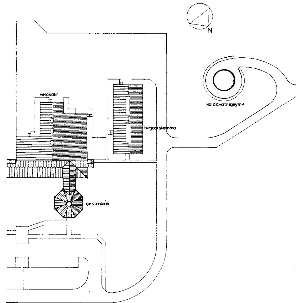
afstöðumynd 1:500
