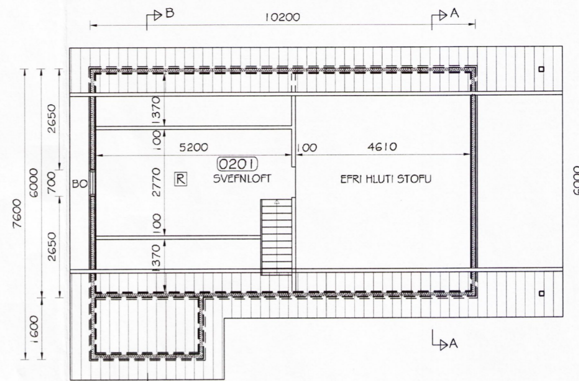
GRUNNMYND EFRI HÆÐAR MKV. 1:100
