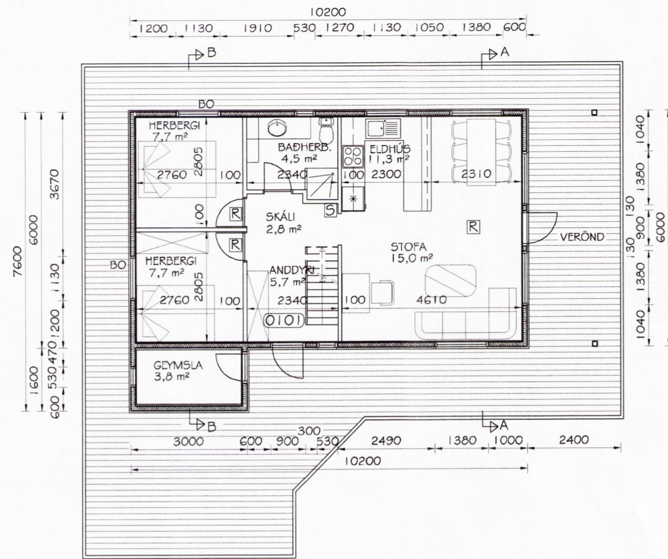
GRUNNMYND MKV. 1:100
