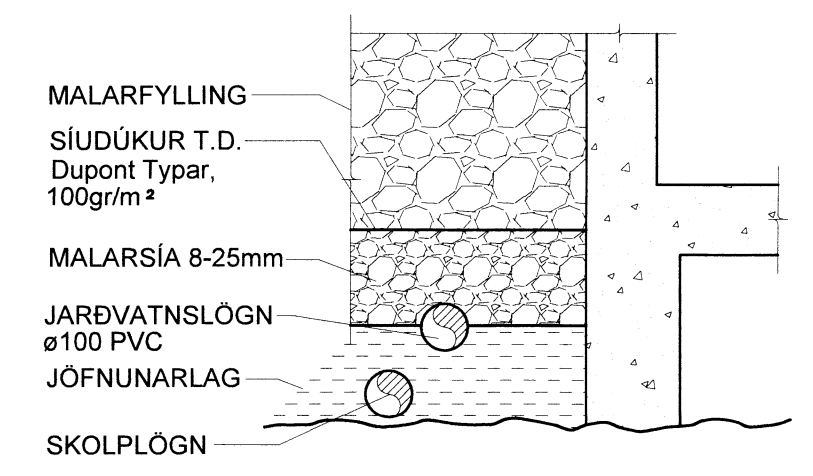
Frágangur jarðvatnslagna úr PVC Mkv. 1:20
