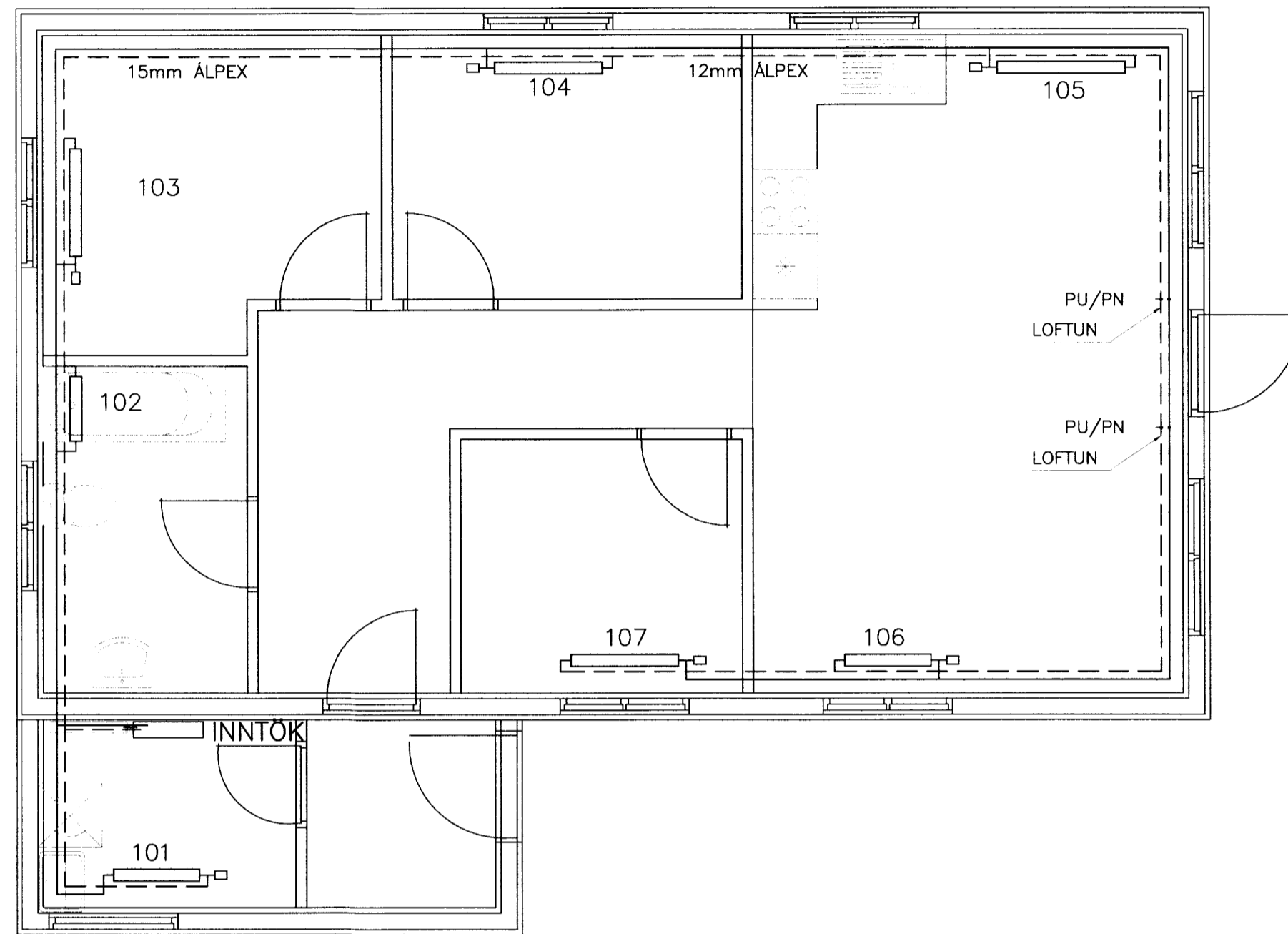
OFNALAGNIR GRUNNMYND MKV. 1:50
