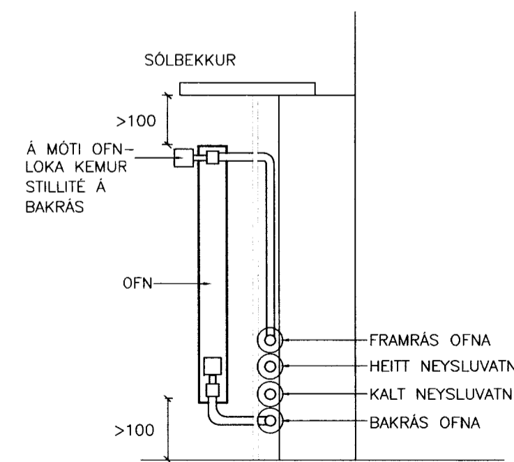
SNID Í VEGG Mkv. 1:10
