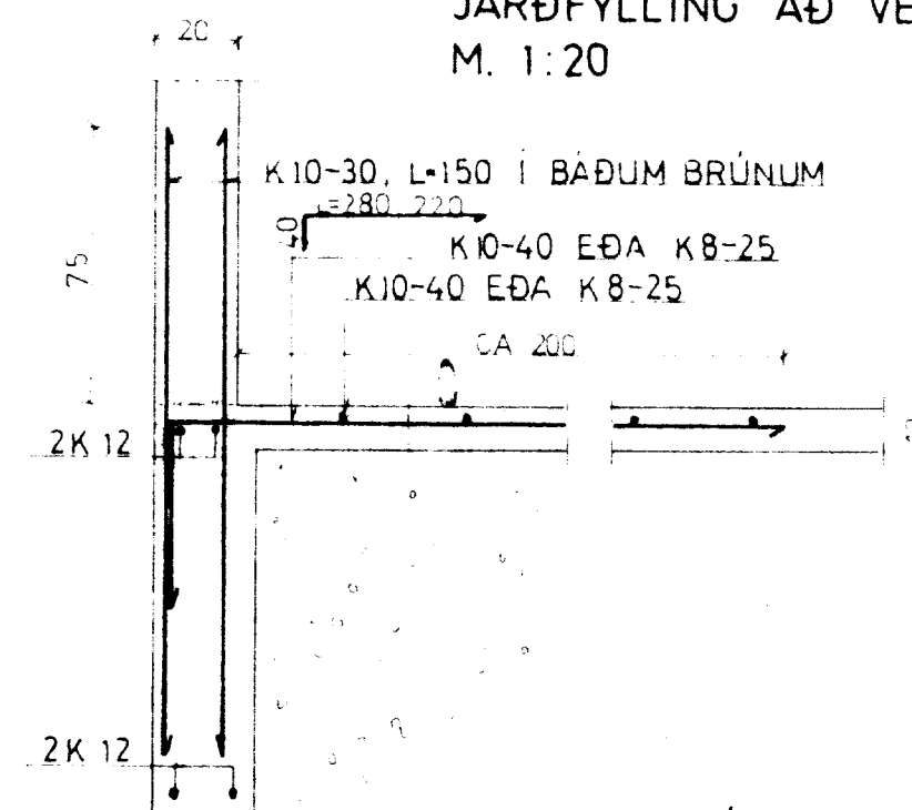
SNID 4-4 HÁIR SÖKKLAR LÍTIL JARÐFYLLING AÐ VEGG M. 1:20
