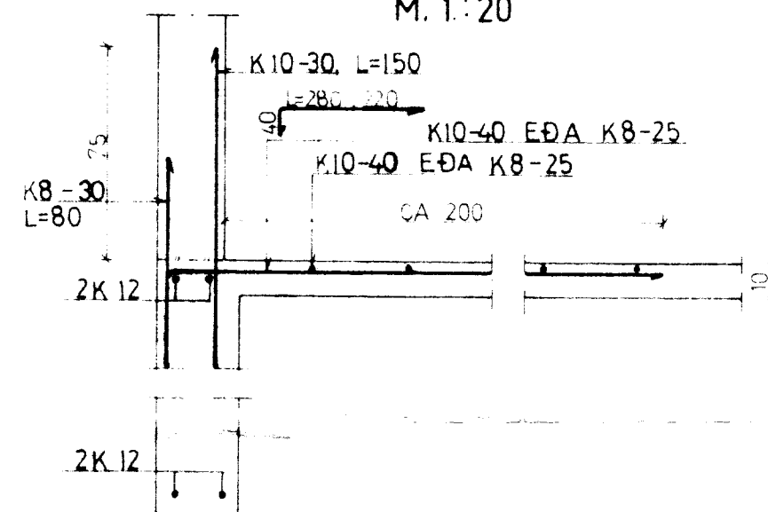
SNID 4-4 HÁIR SÖKKLAR LÍTIL JARÐFYLLING AÐ VEGG M. 1:20
