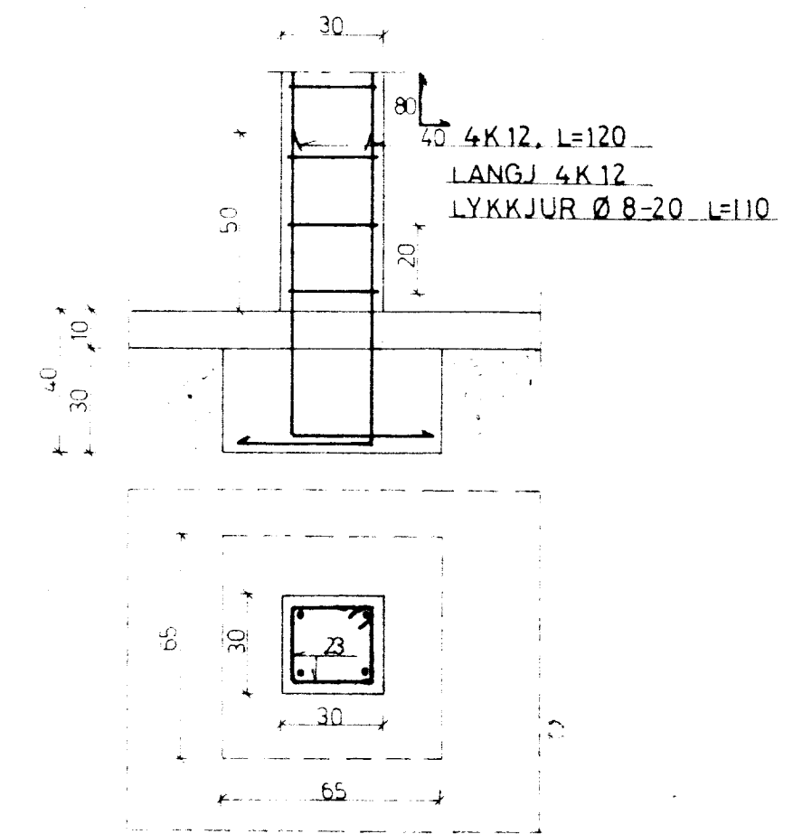
STOÐ MEÐ UNDIRST. M. 1:20
