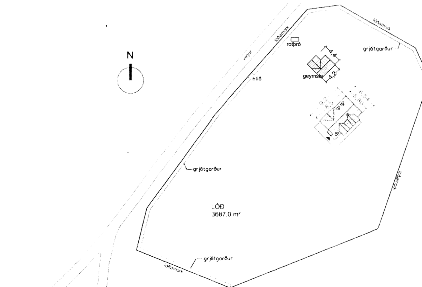
AFSTÖÐUMYND M 1 : 500
