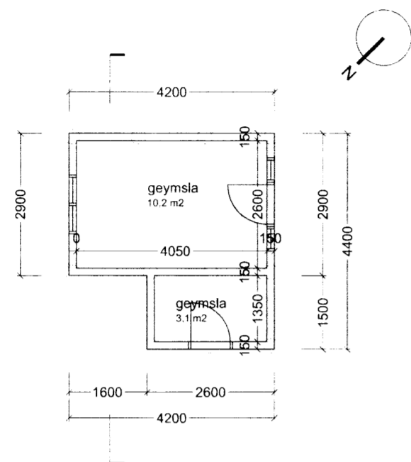
GRUNNMYND M 1 : 100
