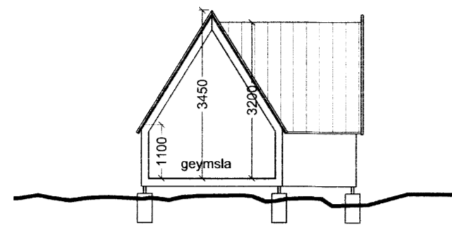
SNEIÐING M 1 : 100
