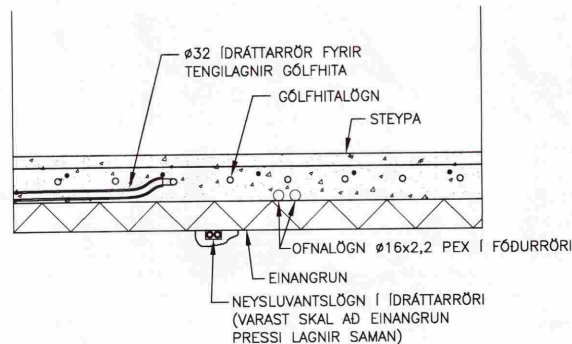
SNIÐ Í GÖLFHITALÖGN Í GRUNNPLÖTU EKKI Í KVARDA
