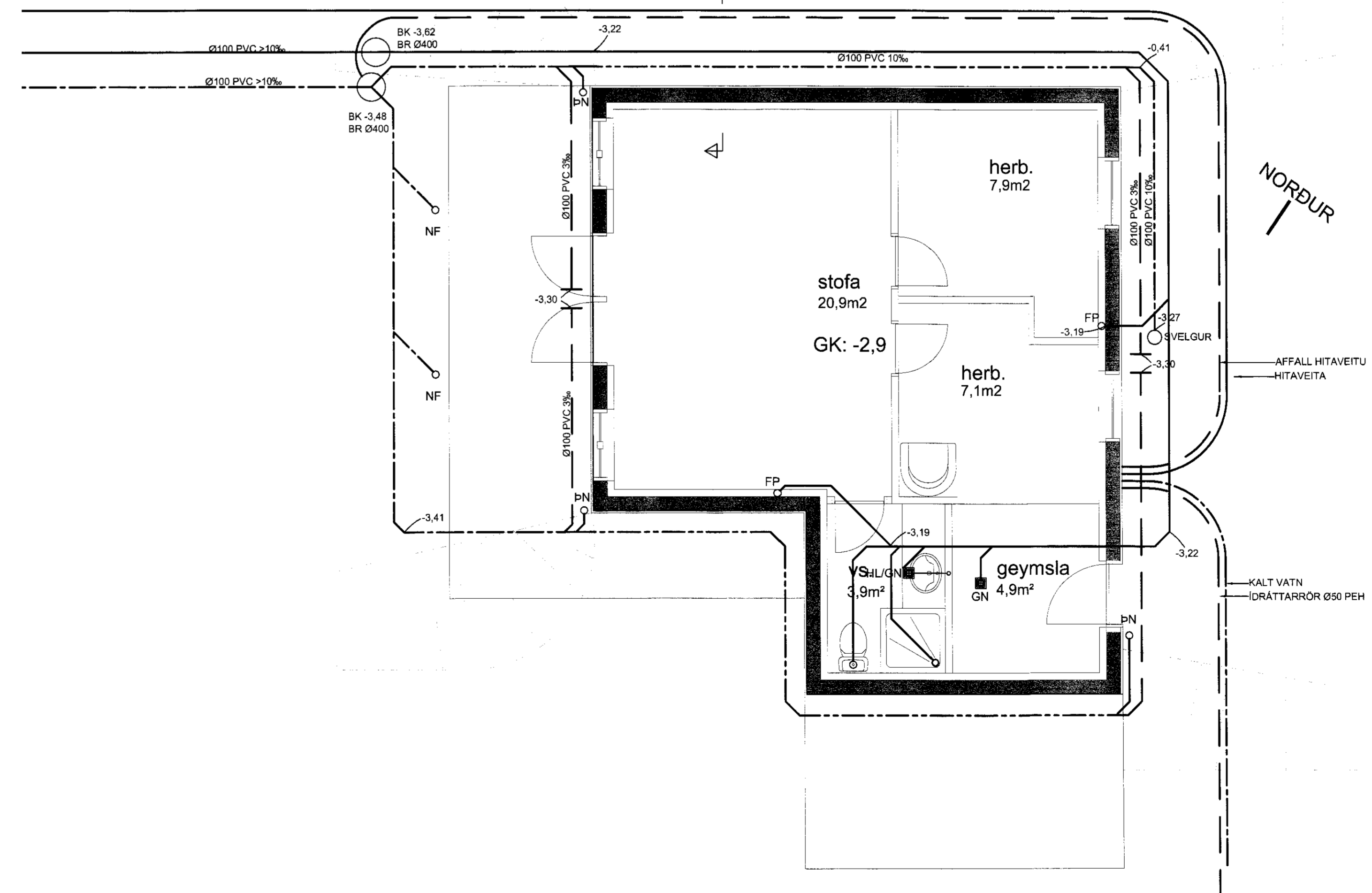
GRUNNMYND 1:50
