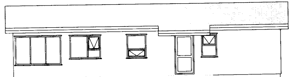
Austur Mkv. 1:100
