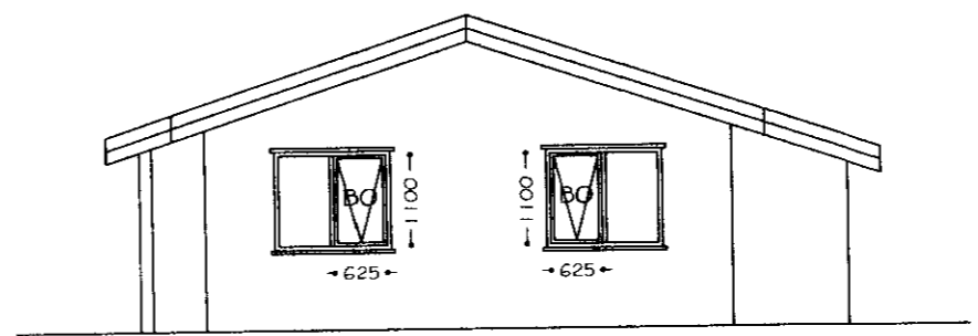
Norður Mkv. 1:100
