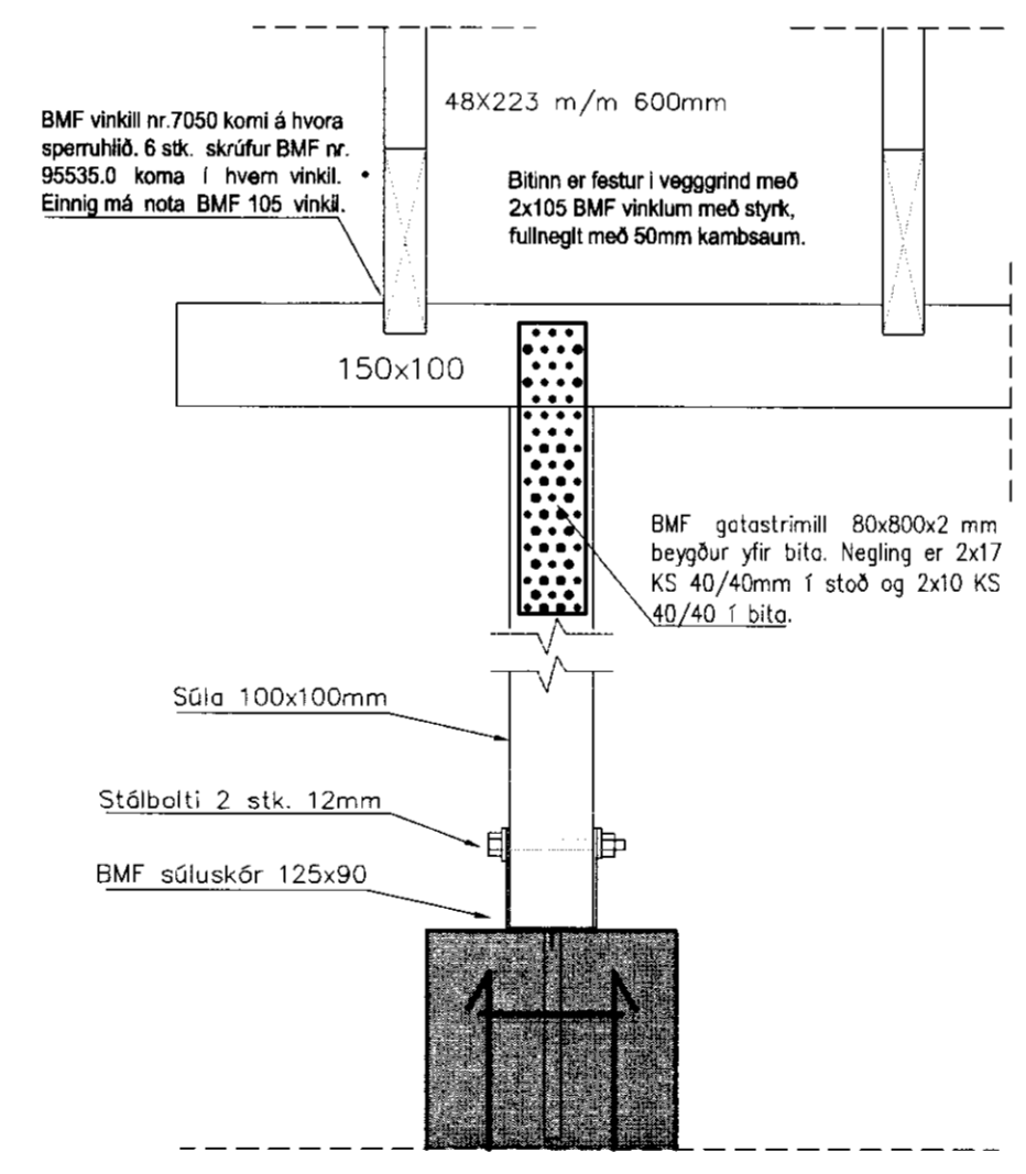
C Snið - Súla í bita 1:10
