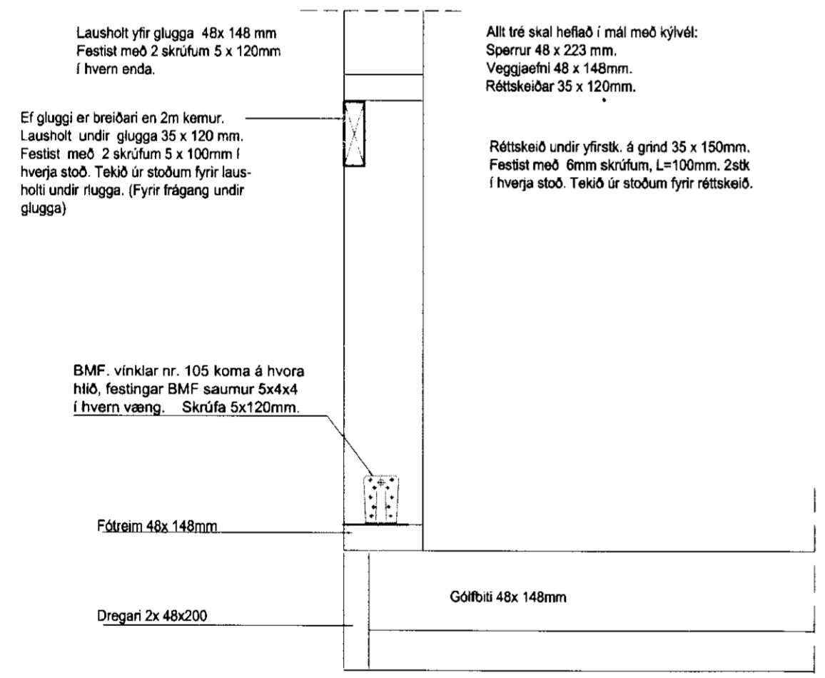
A SNIÐ - Almenn snið í útvegg. Mkv. 1:10
