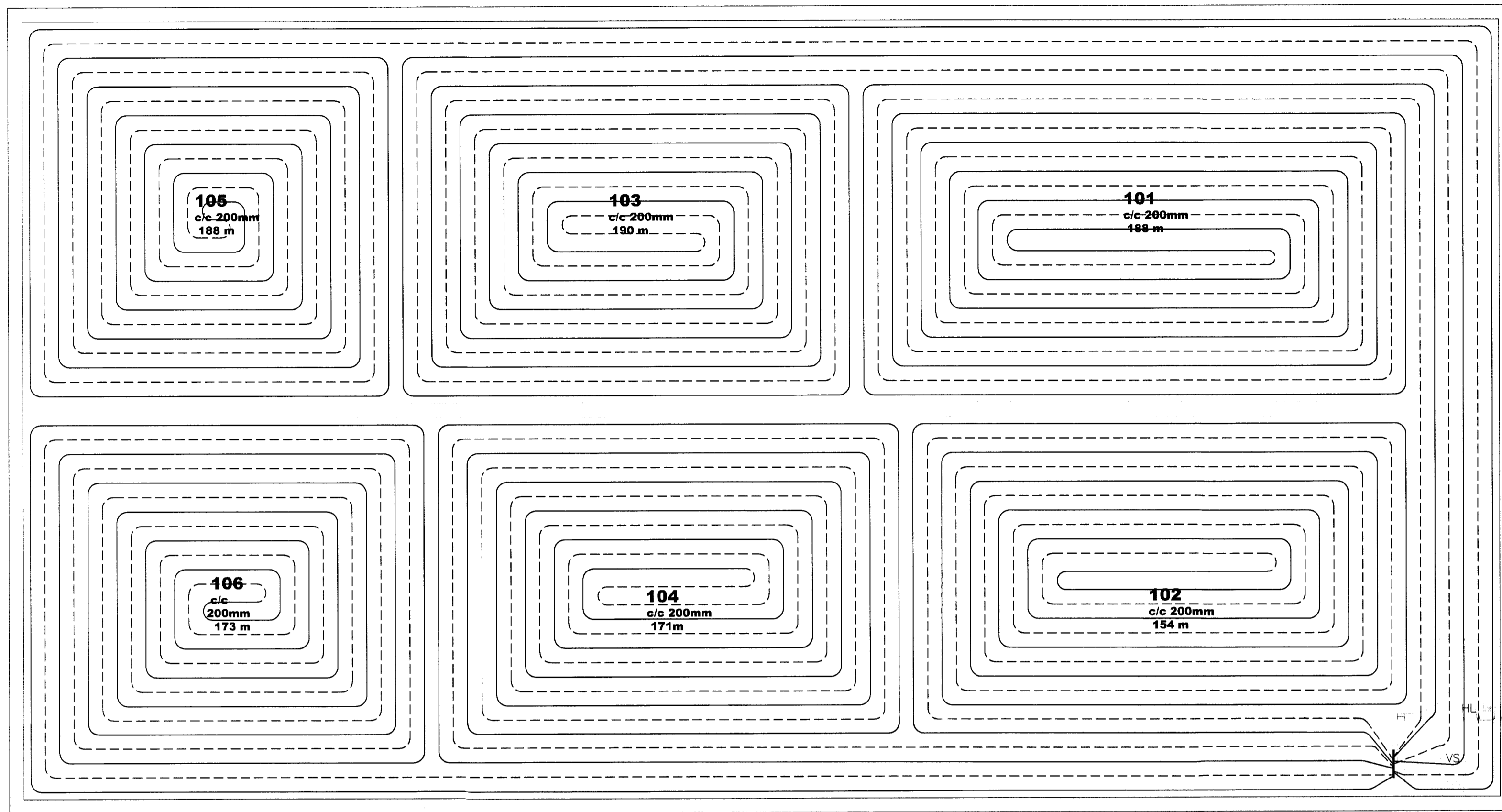
GÓLFHITALAGNIR, GRUNNMYND 1:50
