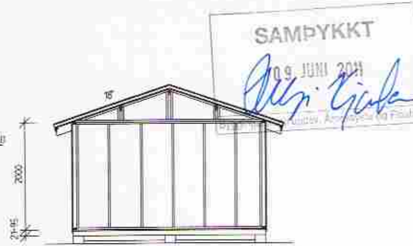
SEKTION SECTION
