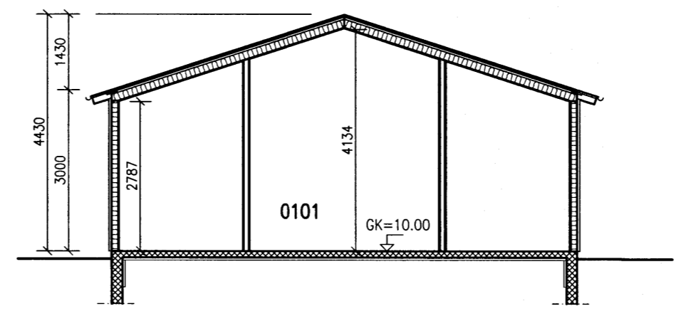
SNID 1-1 1:100
