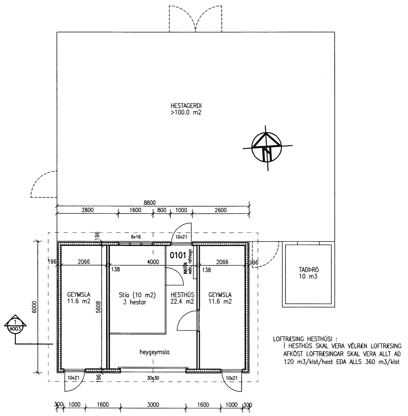
GRUNNMYND 1:100
