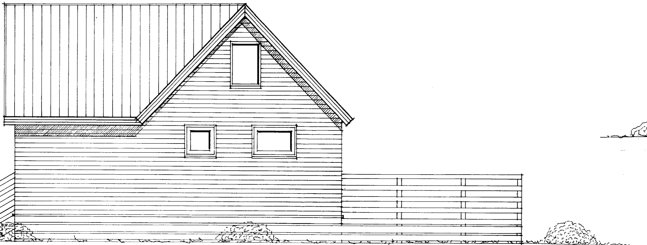
ÚTLIT NORDUR MKV. 1:50
