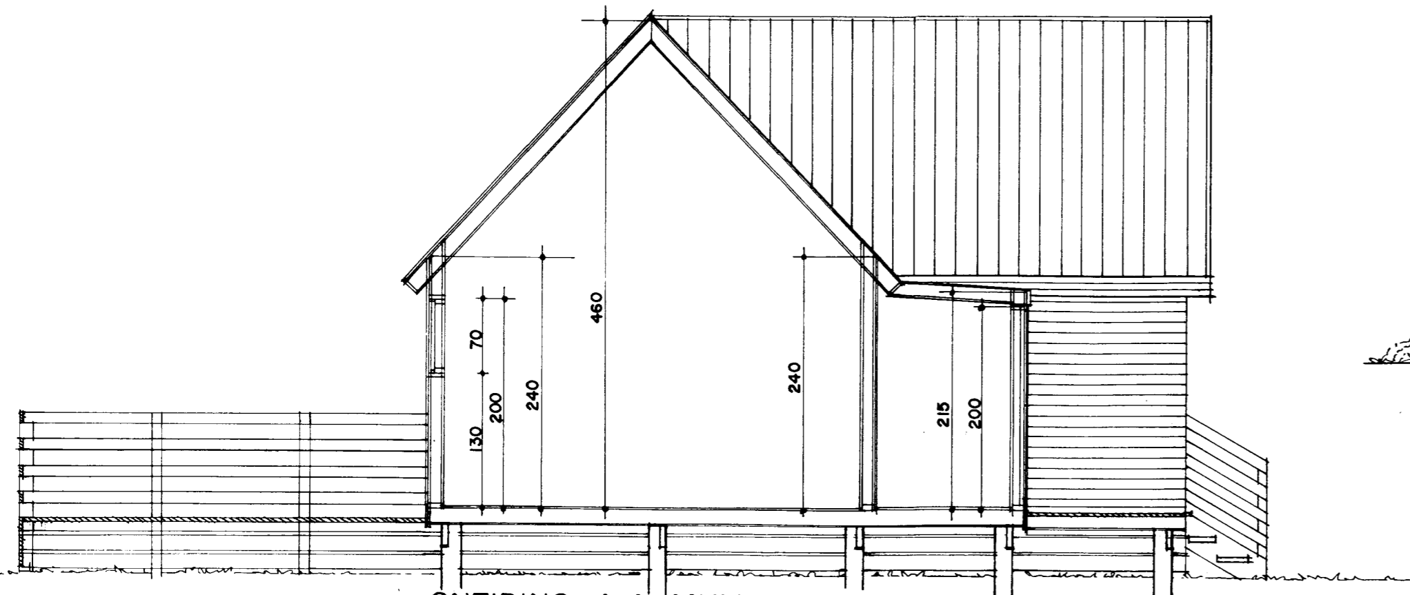
SNEIÐING A-A MKV. 1:50
