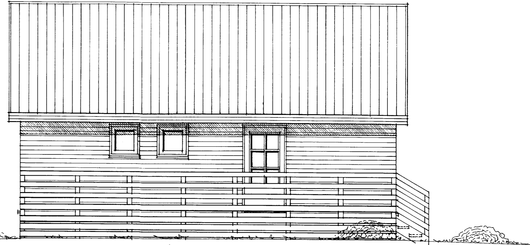
ÚTLIT VESTUR MKV. 1:50
