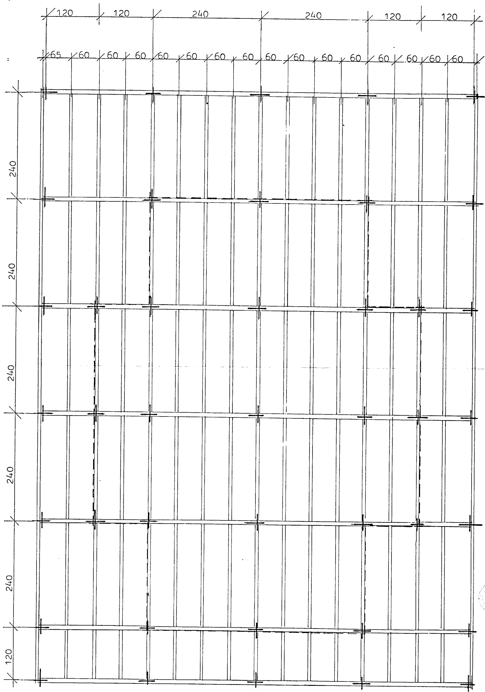
Grunnmynd - gólfbitar og súlur. mkv. 1:50
