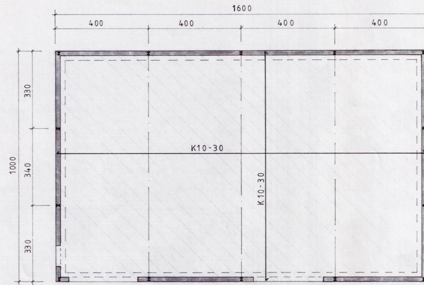
Grunnmynd M=1:100
