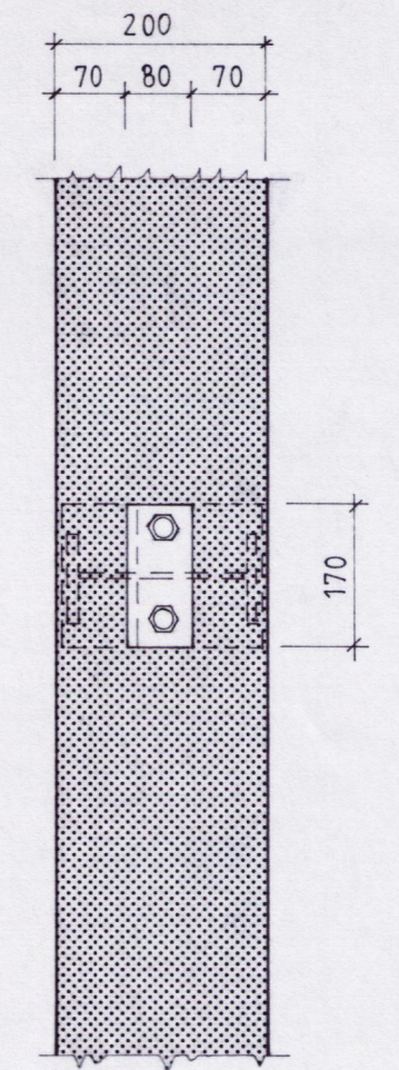
Lár. snið M=1:10
