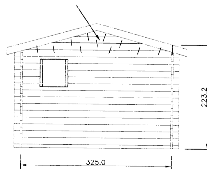
Hliðarmynd gafl festing skásagaðra bjálka
