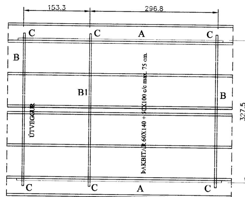
Grunnmynd þak
