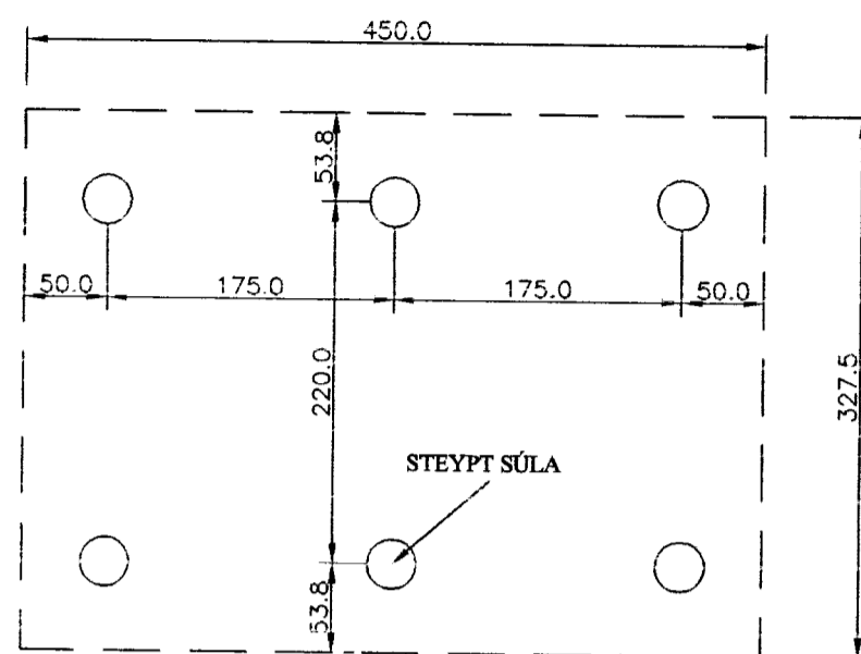
Grunnmynd steypar súlu
