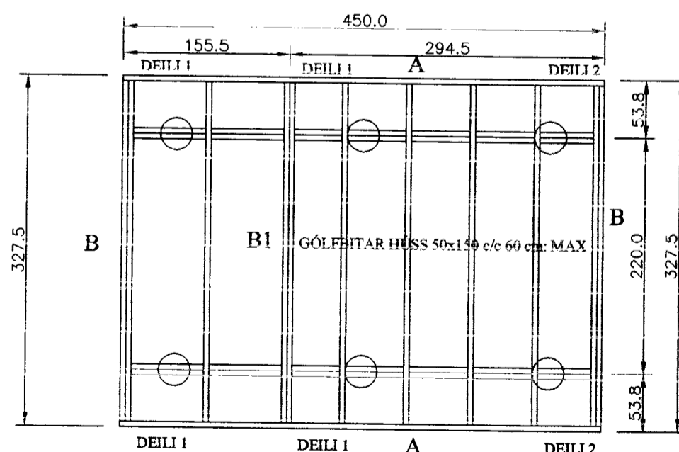
Grunnmynd gólfbitar
