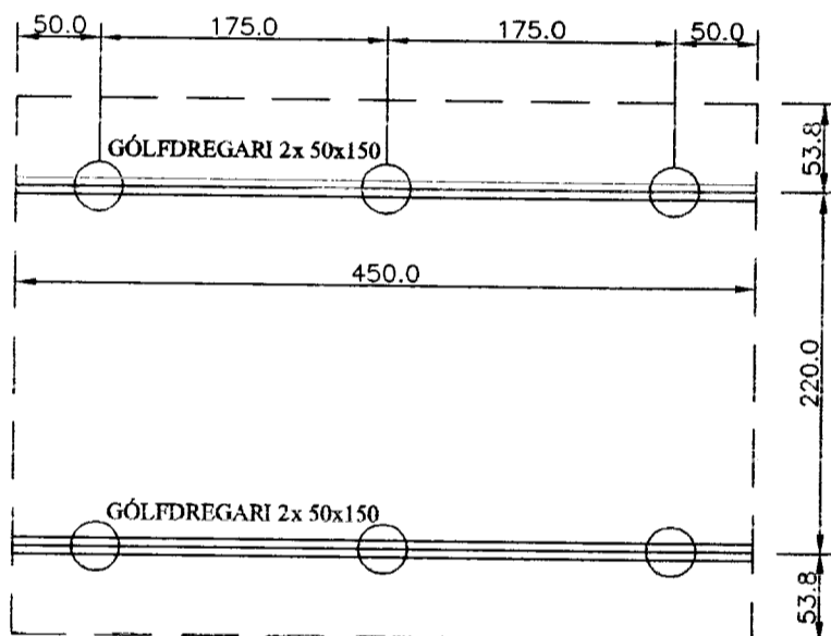
Grunnmynd dregarar
