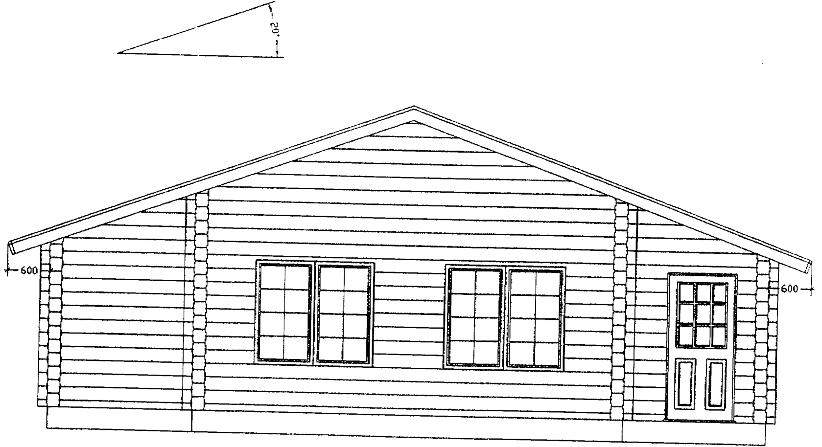
-- FRONT ELEVATION --
