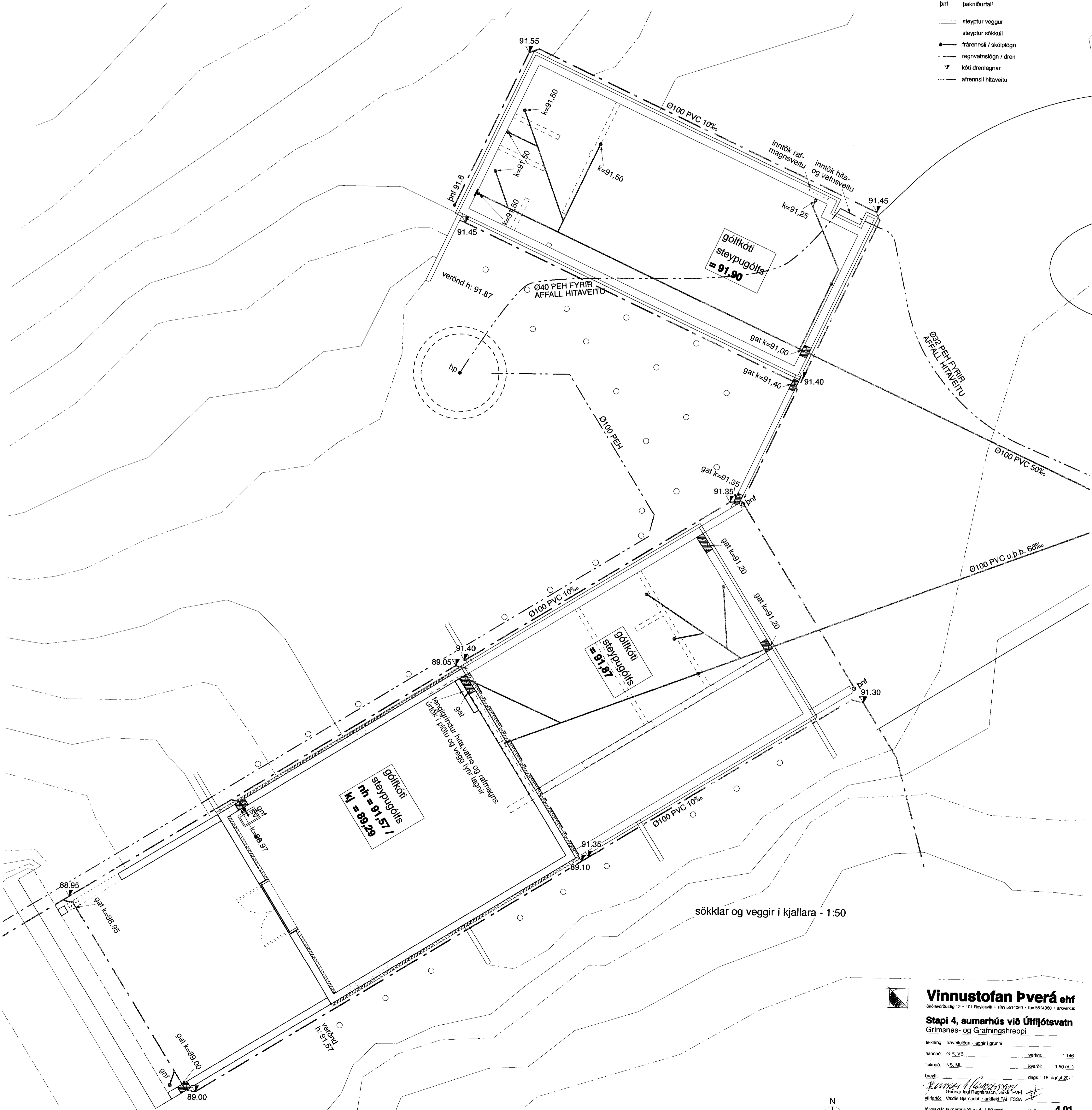
afstöðumynd - 1:500
