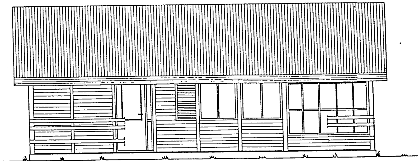
VESTLÆG HLIÐ 1:50
