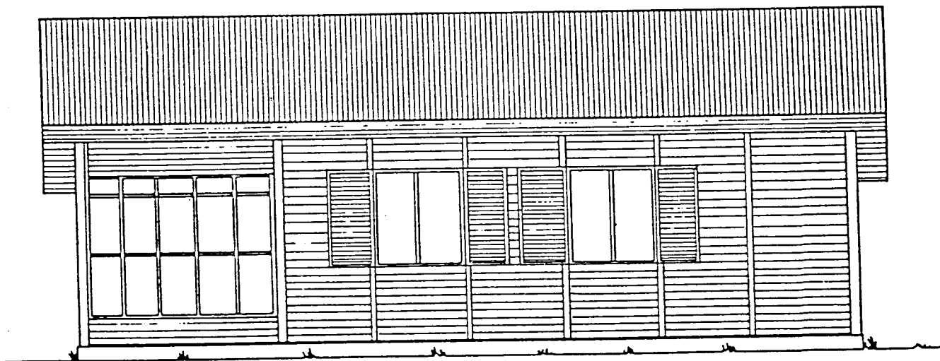
AUSTLÆG HLIÐ 1:50
