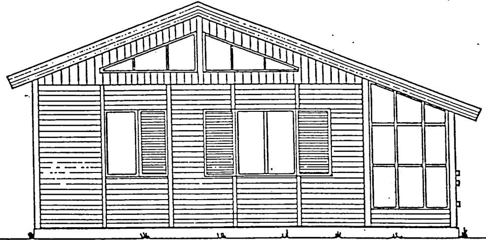
NORÐLÆG HLID 1:50
