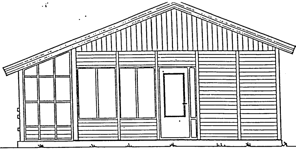
SUDLÆG HLID 1:50
