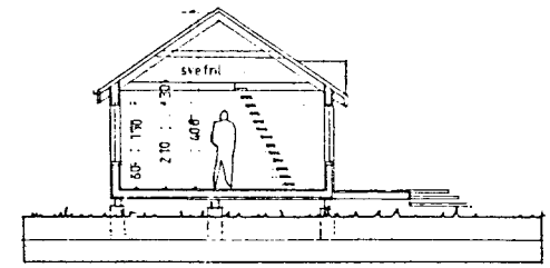
sneiding mkv. 1:100
