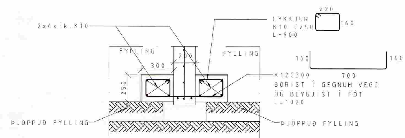
BREYTING Á SÖKKULFÓT 1:20 UNDIR MIÐVEGGJUM SJÁ GRUNNMYND
