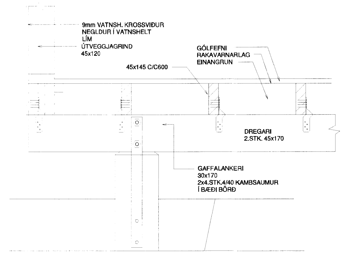
SNID B-B 1:10
