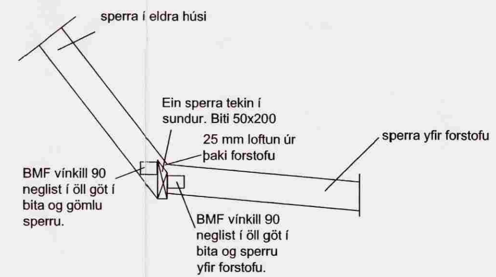
snið B 1:20 (blað nr. S-04) samsetning sperru yfir forstofu og eldra húss
